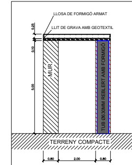
SECCIÓ A - A
