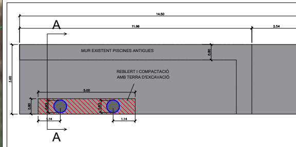
PLANTA DE FONAMENTACIÓ
