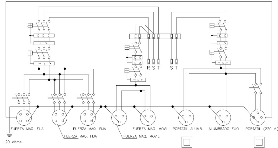
ESQUEMA UNIFILAR DEL CUADRO ELECTRICO DE OBRA
