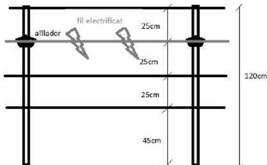
Detall del tipus de tancament
