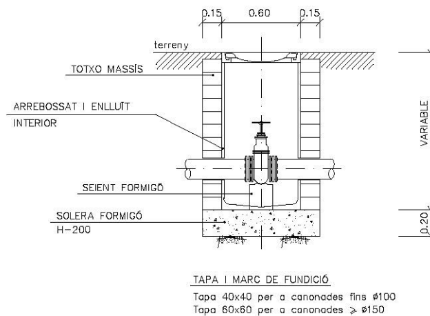
Fig. Arqueta tipus per vàlvula de tall
