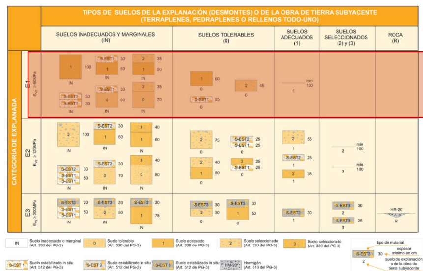
FIGURA 1. FORMACIÓN DE LA EXPLANADA
