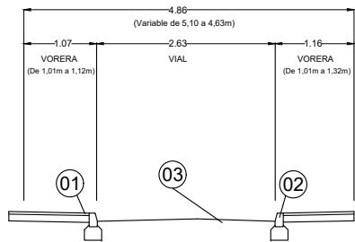
CARRER CASTELLET (PLAÇA D'ANSELM CLAVÉ - CARRER GRAN)
