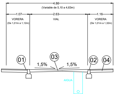
CARRER CASTELLET (PLAÇA D'ANSELM CLAVÉ - CARRER GRAN)
