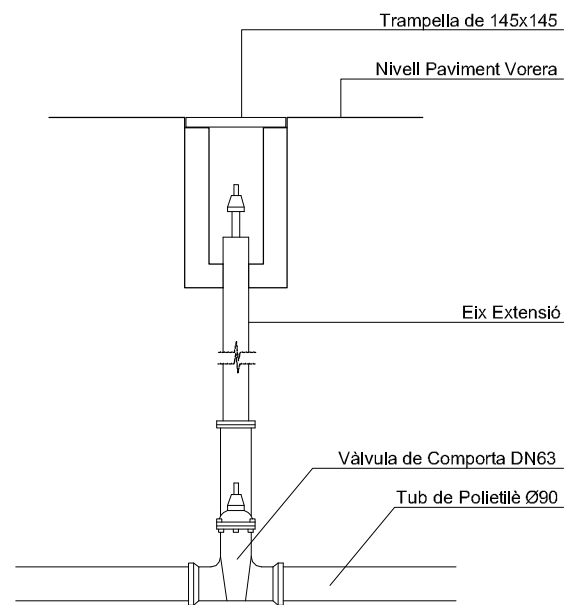
Troneta tipus II (Clau de pas) e. 1/20
