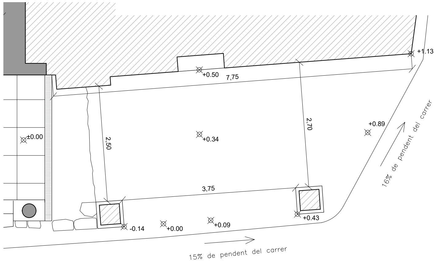
PLANTA ACTUAL
