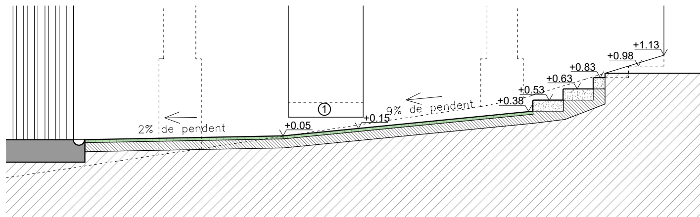
SECCIÓ PROPOSTA
