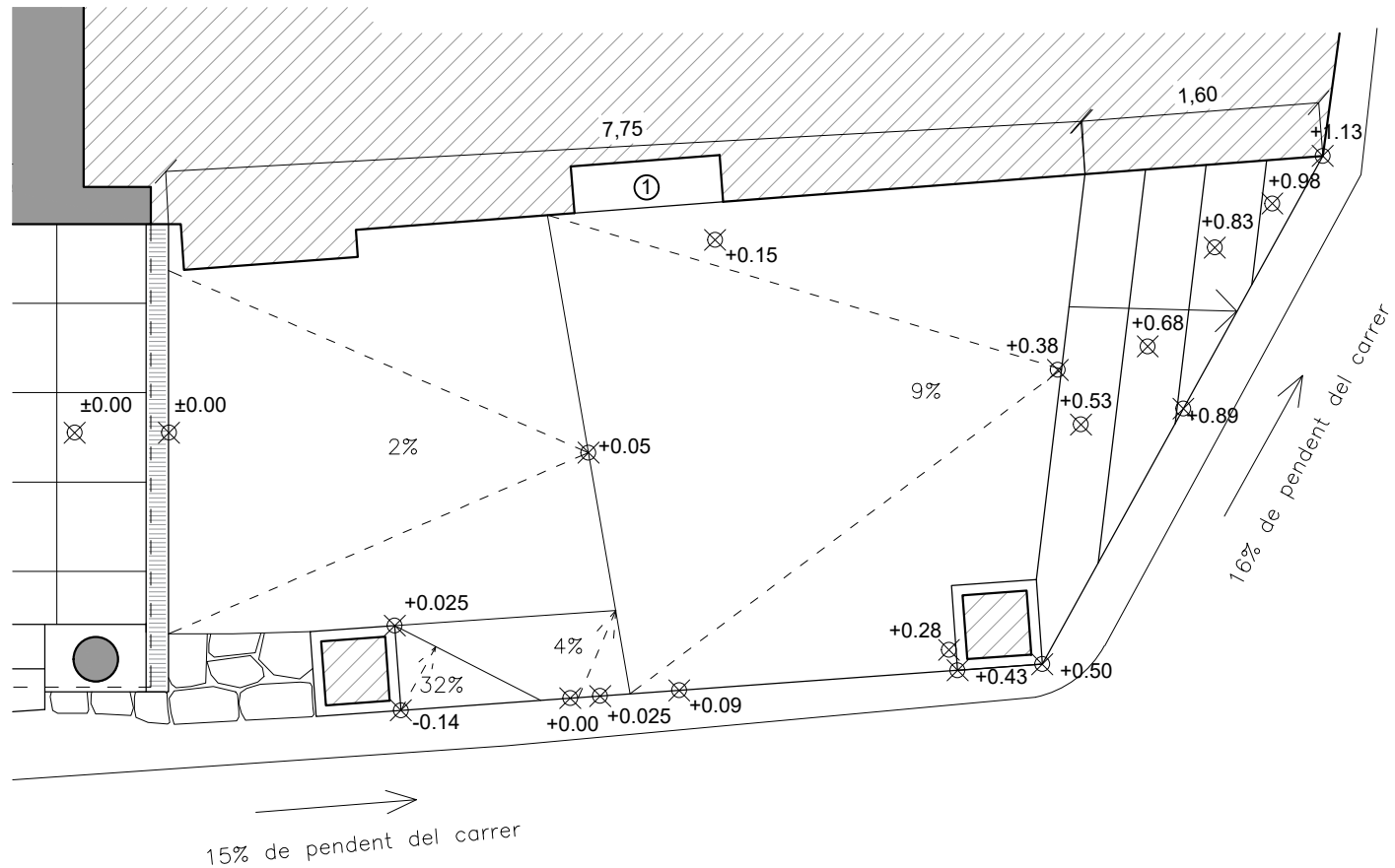
PLANTA PROPOSTA
