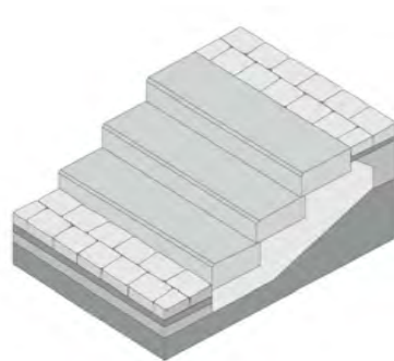
Detall graons prefabricats de formigó.
