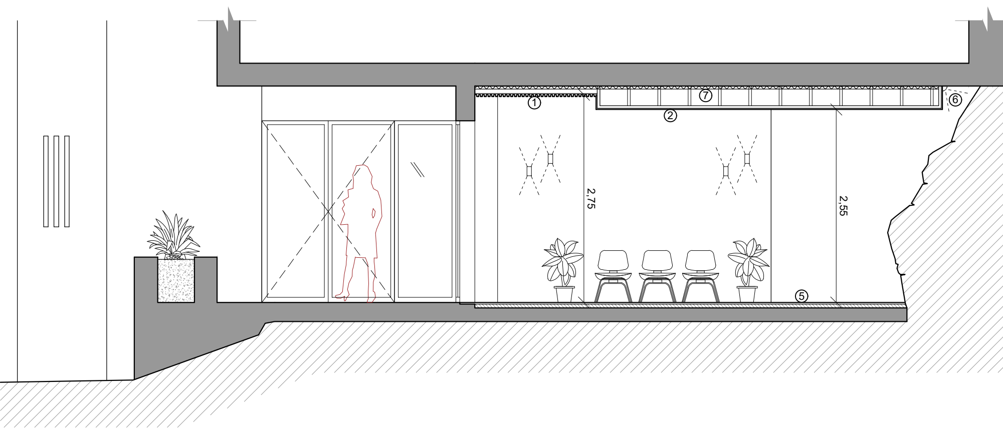
SECCIÓ B-B'
