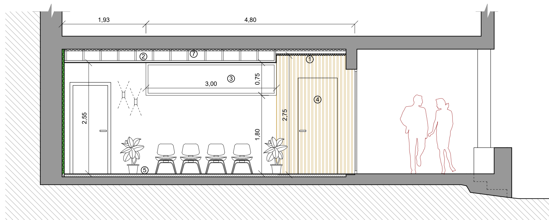
SECCIÓ A-A'
