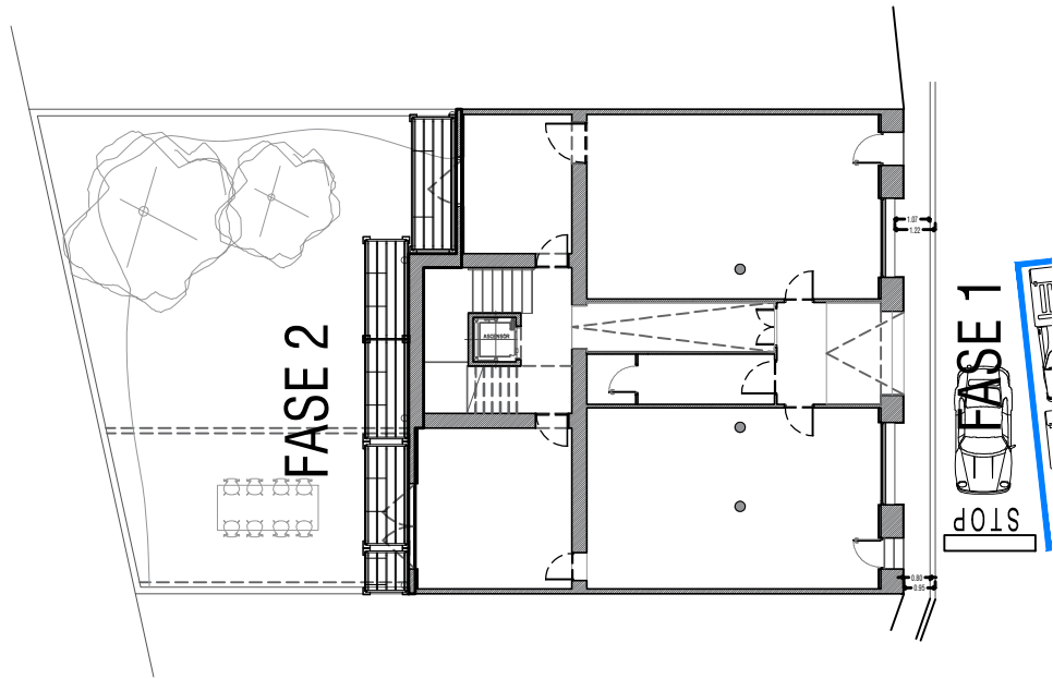
PLANTA BAIXA
