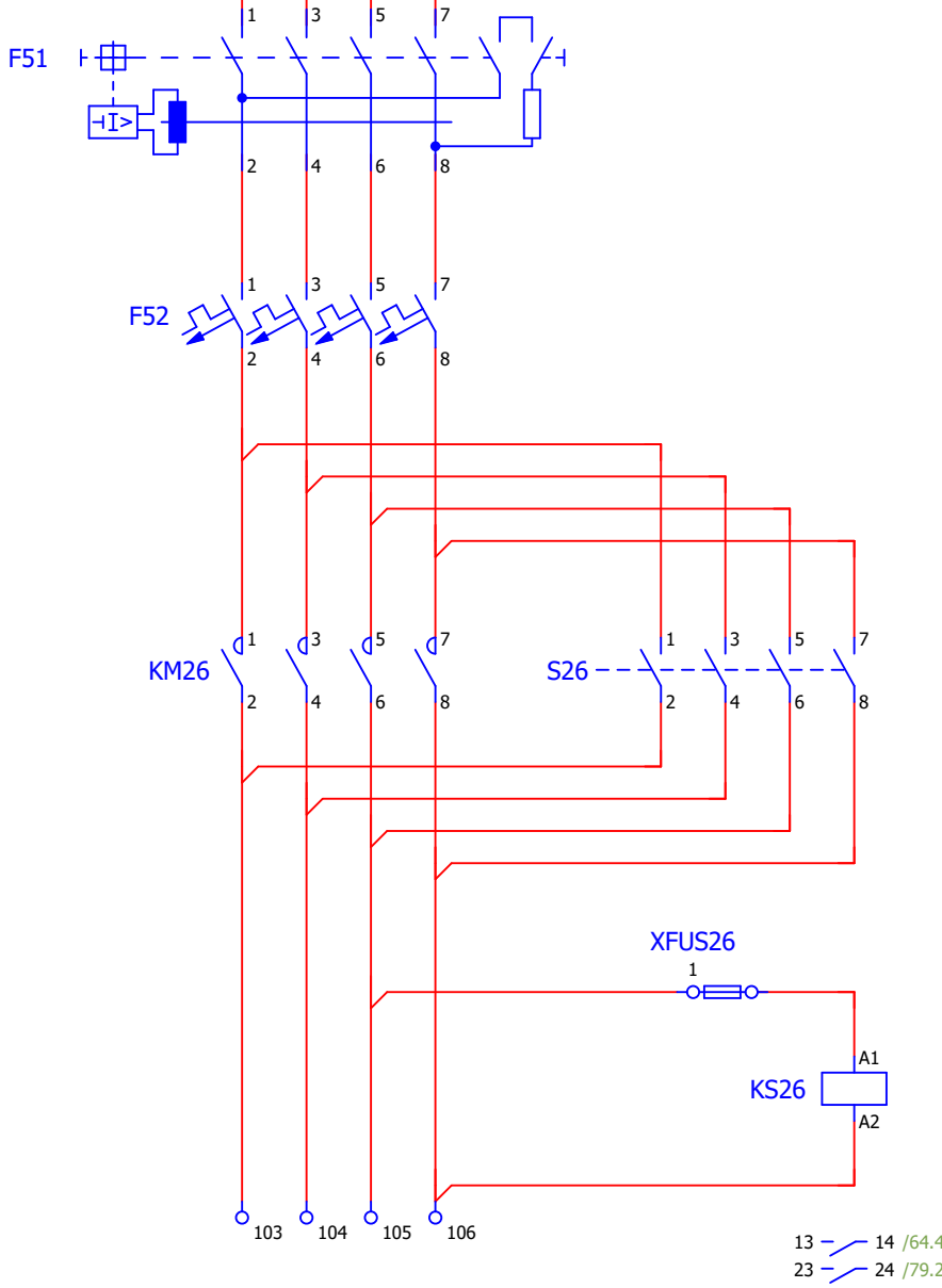
Circuit ennuolat 2
