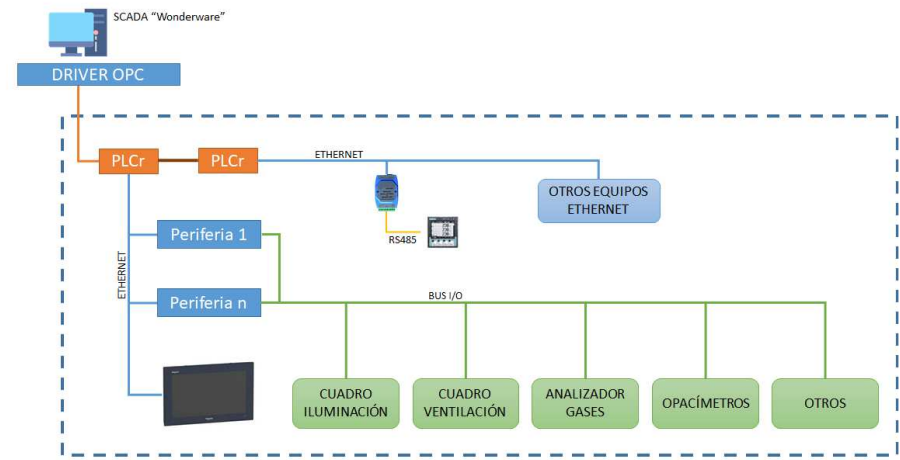
SOLUCIÓN TÚNEL LARGO (SISTEMA REDUNDADO)
