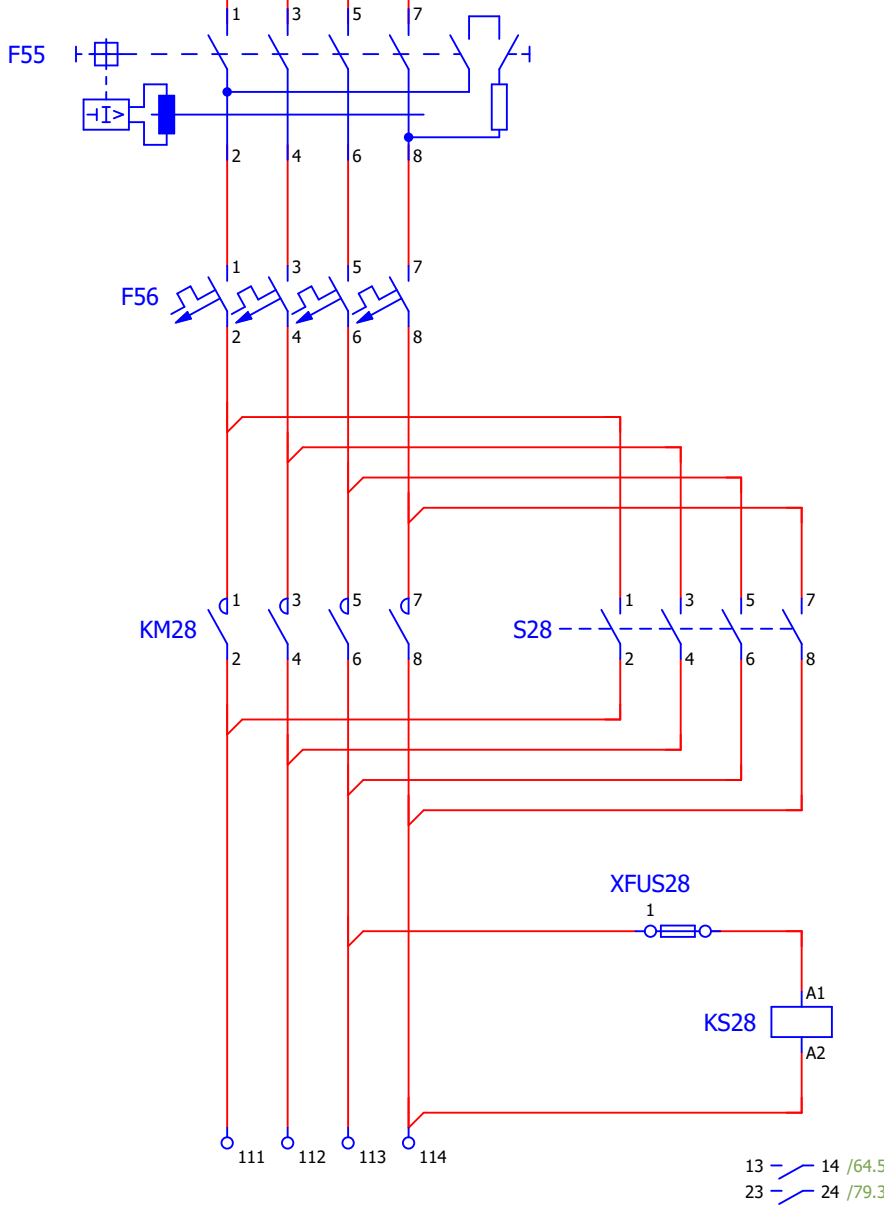
Circuit ennuolat 4
