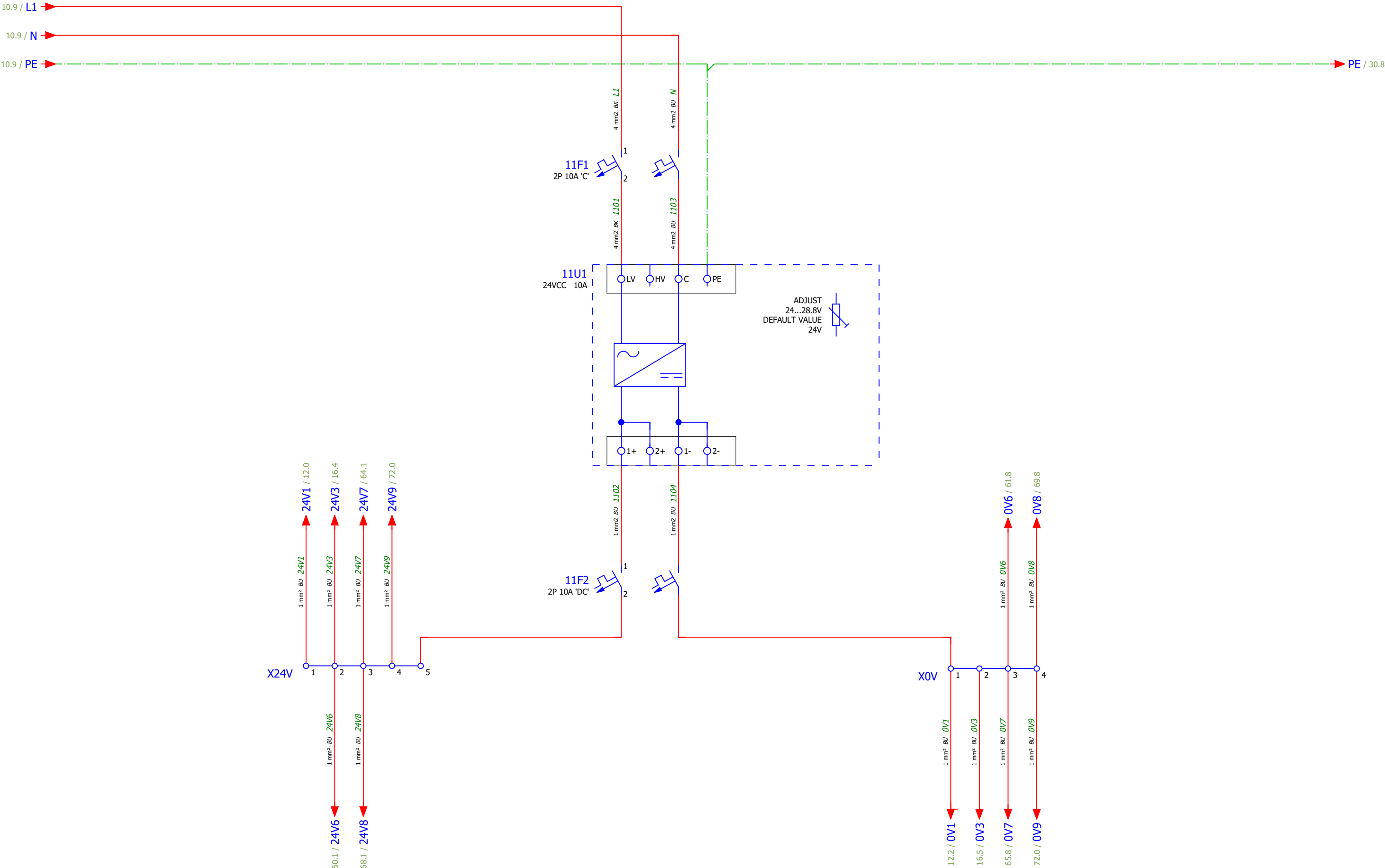
Fuente alimentación
