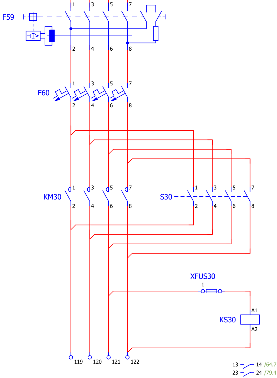
Circuit ennuolat 6
