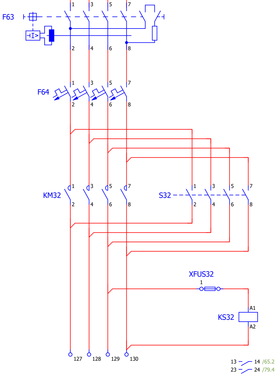
Circuit ennuolat 8
