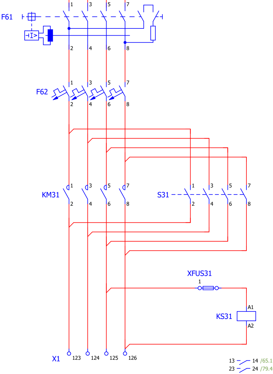
Circuit ennuolat 7
