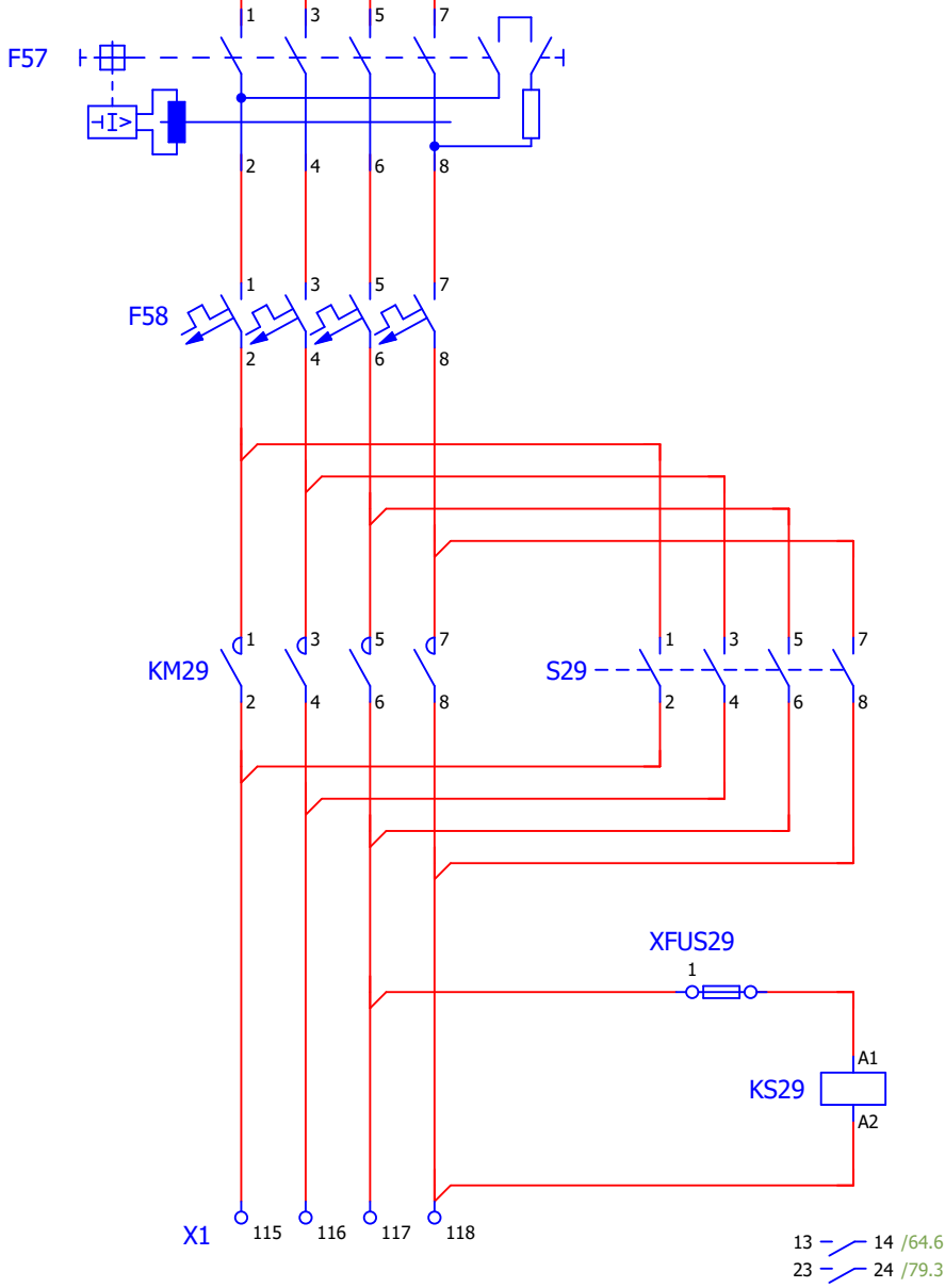
Circuit ennuolat 5
