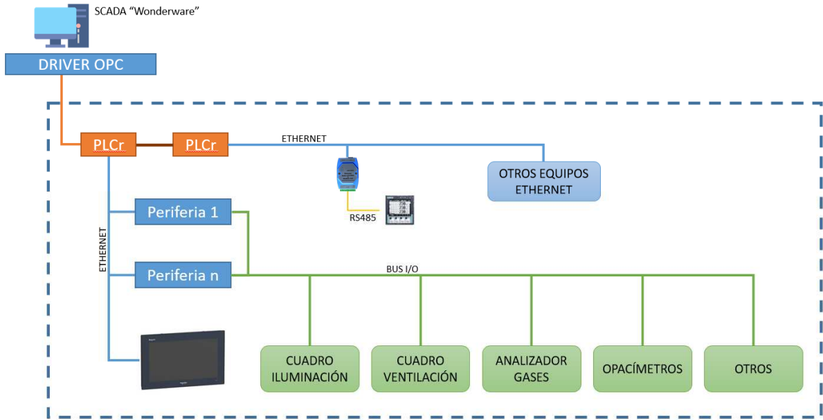
SOLUCIÓN TÚNEL LARGO (SISTEMA REDUNDADO)
