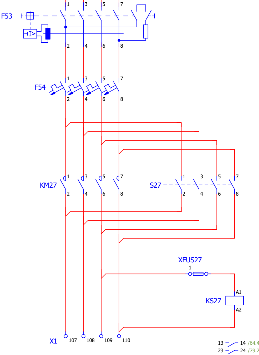
Circuit ennuolat 3
