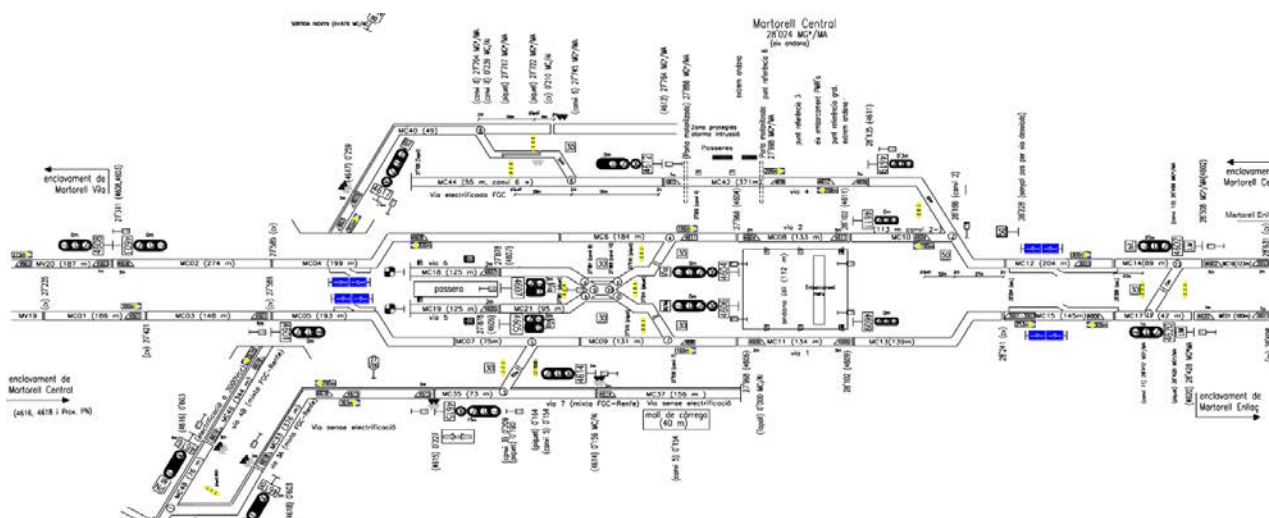
Fig. 4: Esquema de vies de l'àmbit de l'enclavament de Martorell Central
