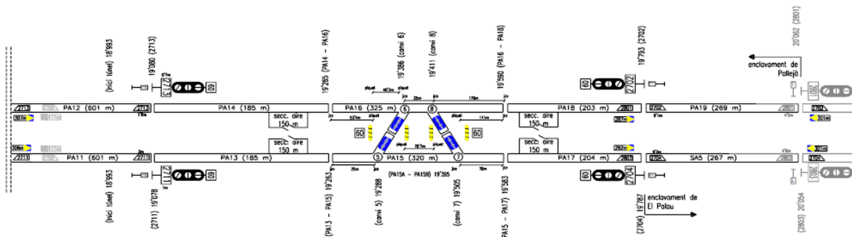
Fig. 1: Esquema de vies de l'àmbit de l'enclavament de Pallejà
