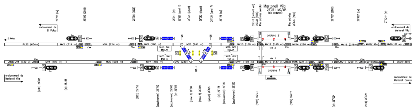
Fig. 3: Esquema de vies de l'àmbit de l'enclavament de Martorell Vila
