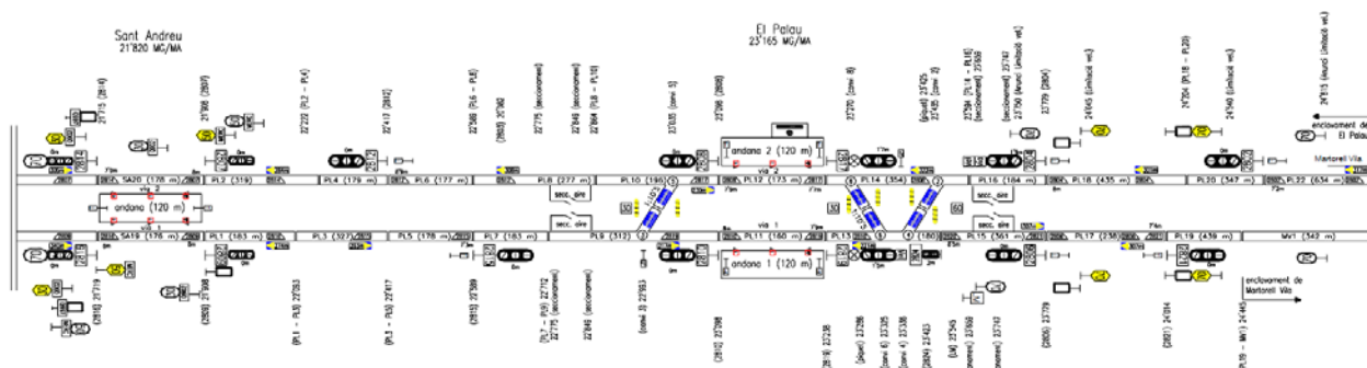
Fig. 2: Esquema de vies de l'àmbit de l'enclavament de El Palau
