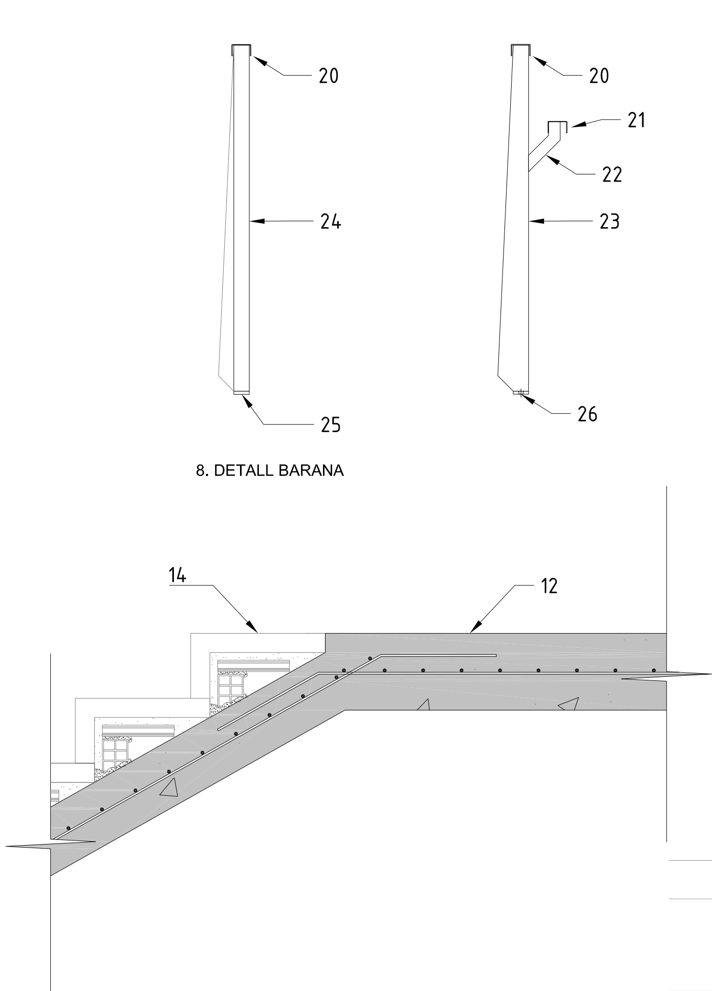
5. ARRENCADA D'ESCALA
