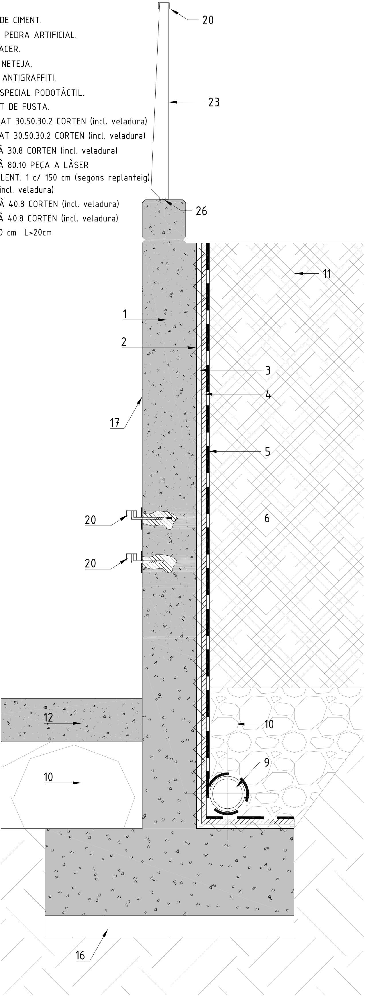
1. DETALL SECCIÓ MUR TIPUS
