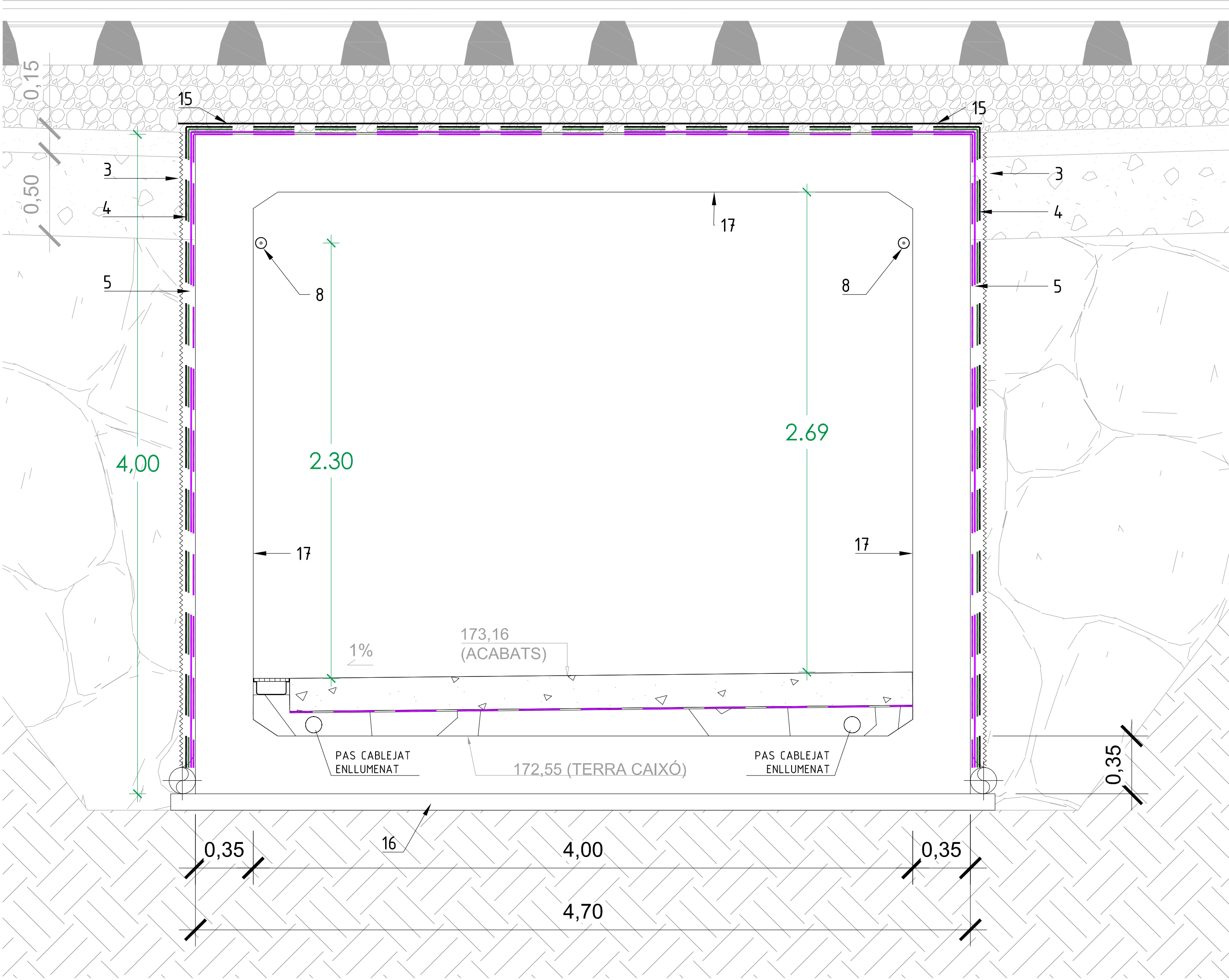
3. DETALL PAS SOTERRAT VIANANTS
