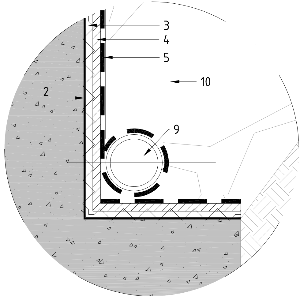
2. DETALL TUB DREN
