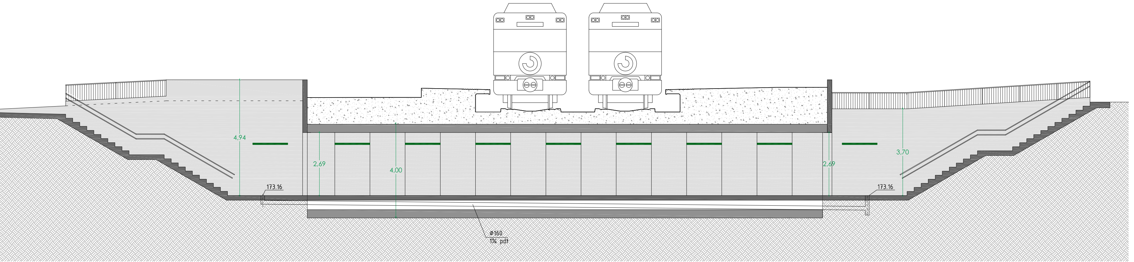
SECCIÓ C-C'
