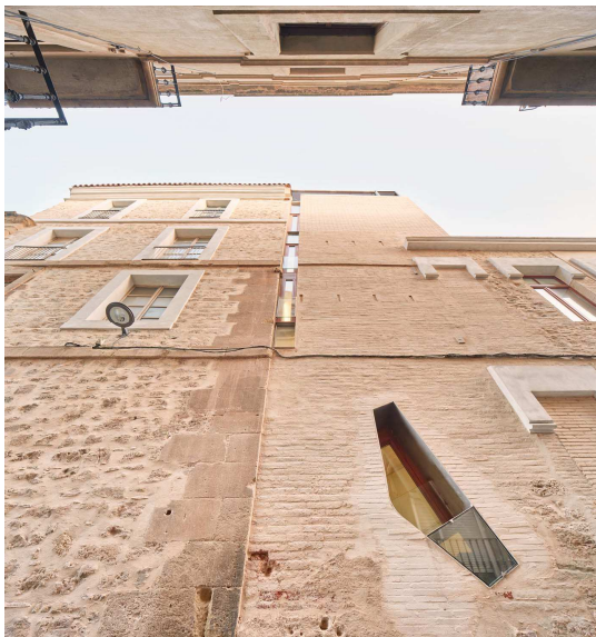
Rehabilitació de la façana sud amb el volum del nucli del muntacàrregues
