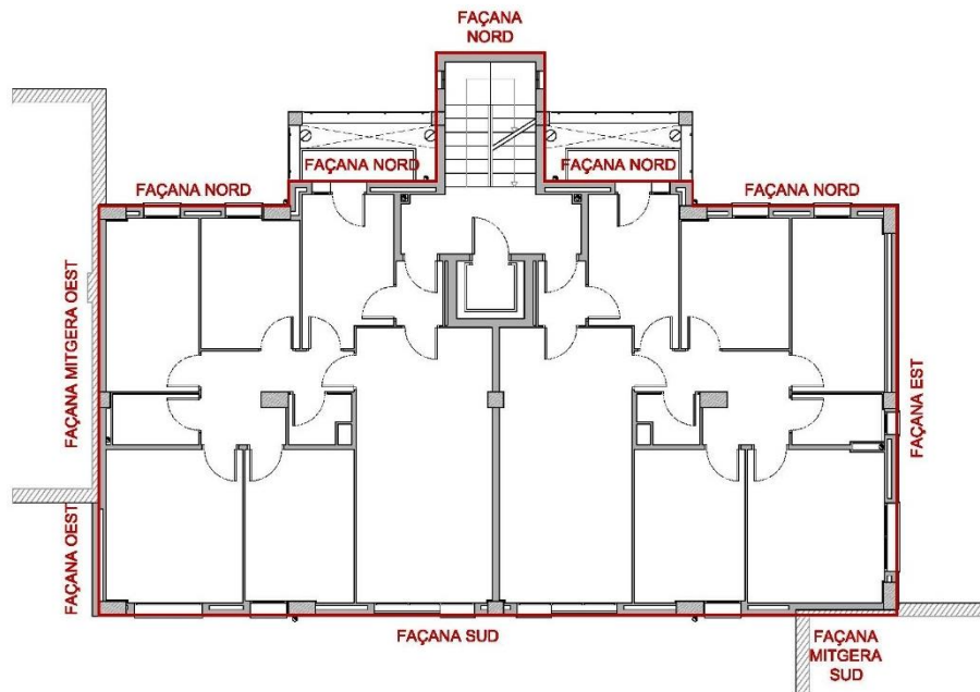
*Planta tipus de l'edifici 8B.
