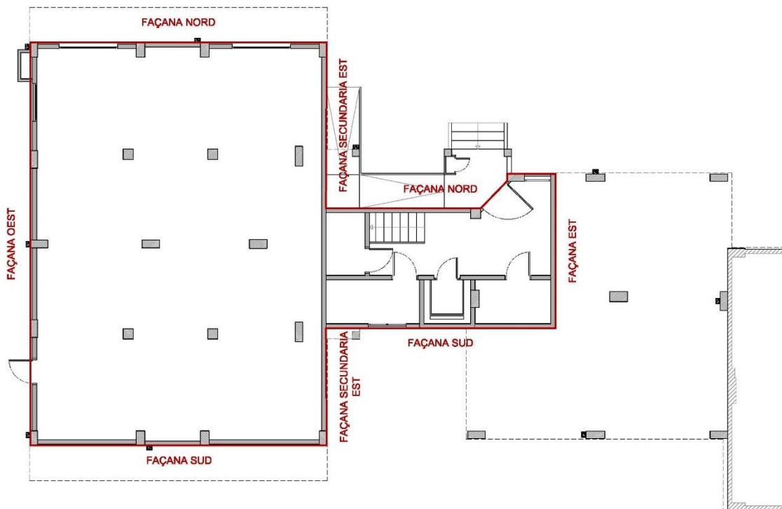
*Planta baixa de l'edifici 8A.
