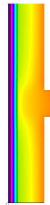
*Càlcul ponts tèrmics amb zones tèrmiques.
