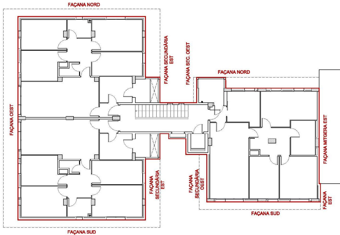
*Planta tipus de l'edifici 8H.
