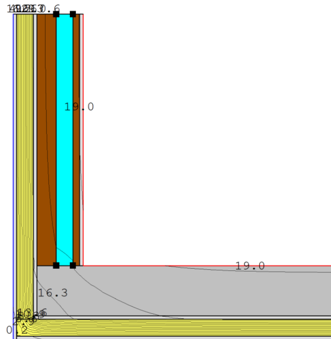
*Càlcul ponts tèrmics amb Isolinies.
