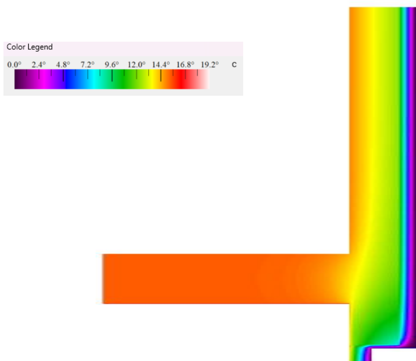
*Càlcul ponts tèrmics amb zones tèrmiques.
