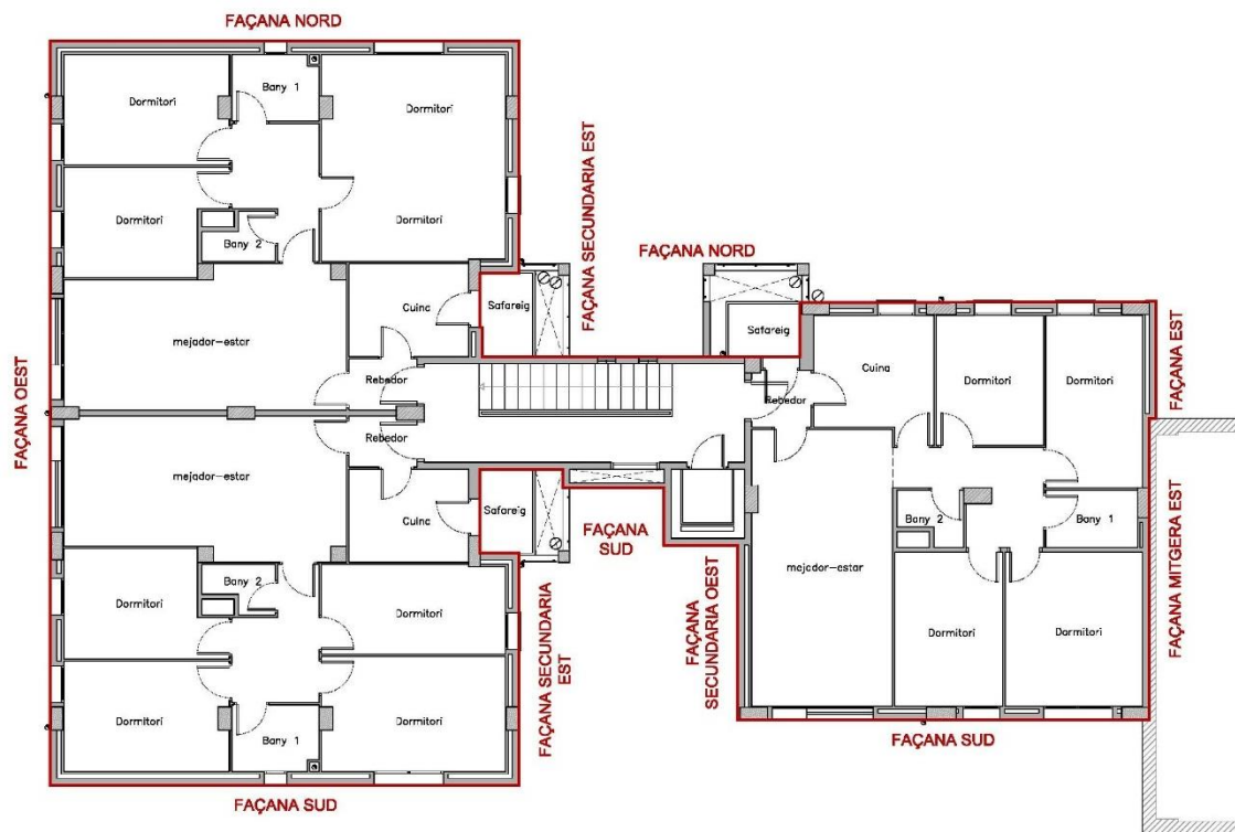
*Planta tipus de l'edifici 8A.
