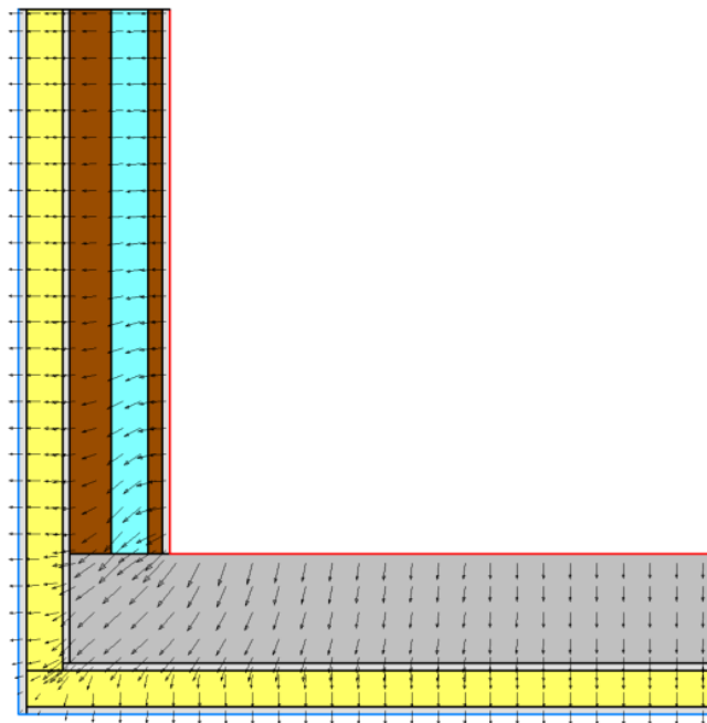
*Càlcul ponts tèrmics amb vectors de fluxe.
