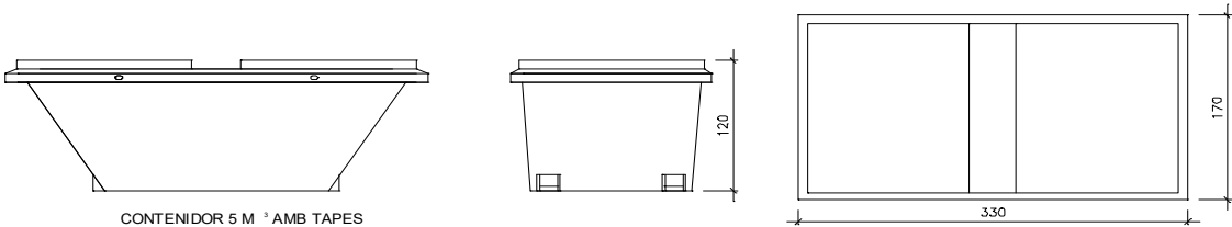
Contenedor 5 m³. Apte per a plàstics, paper i cartro, metalls i fusta
