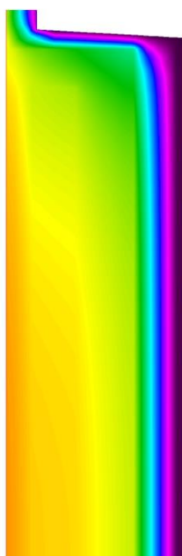
*Càlcul ponts tèrmics amb zones tèrmiques.
