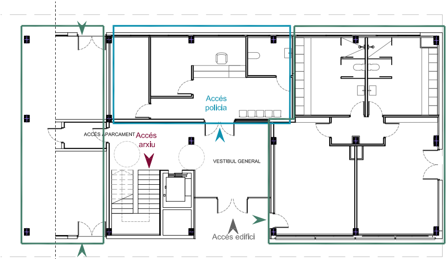
PLANTA BAIXA
