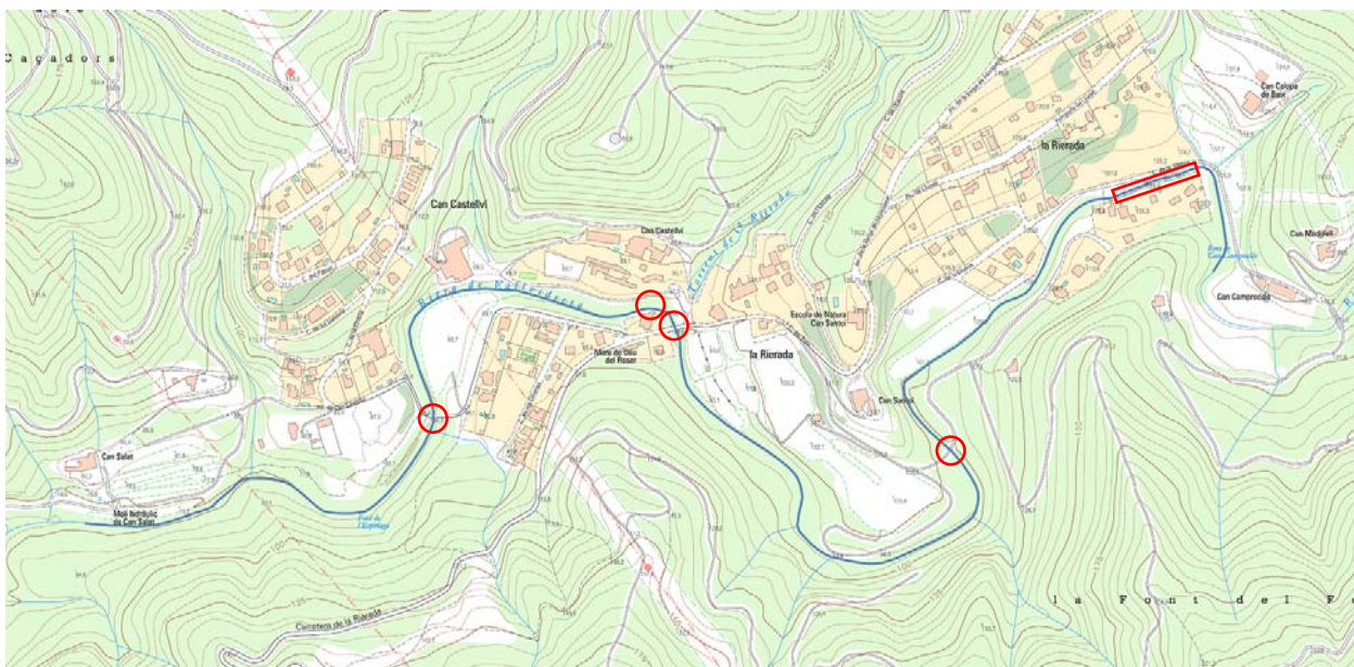
Figura 5 Ponts i passeres existents
