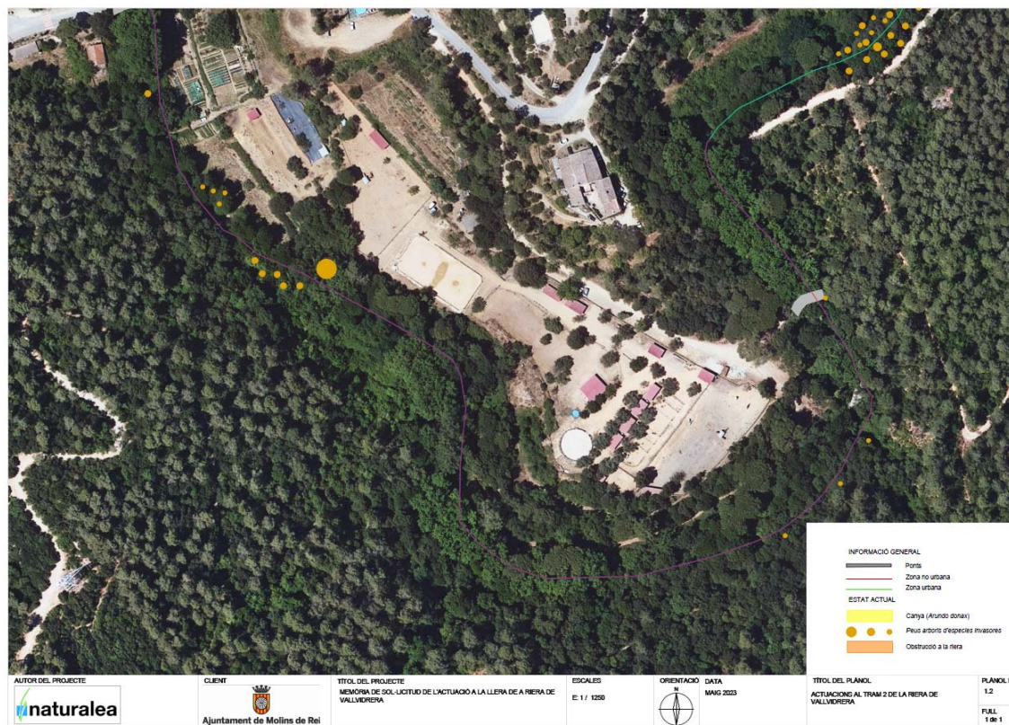
Figura 16 Plànol de les actuacions al tram en zona no urbana del projecte
