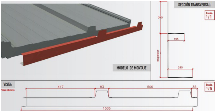
Detall muntatge frontal panell
