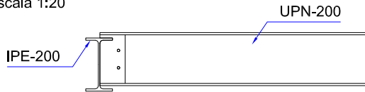
Detall B Escala 1:20
