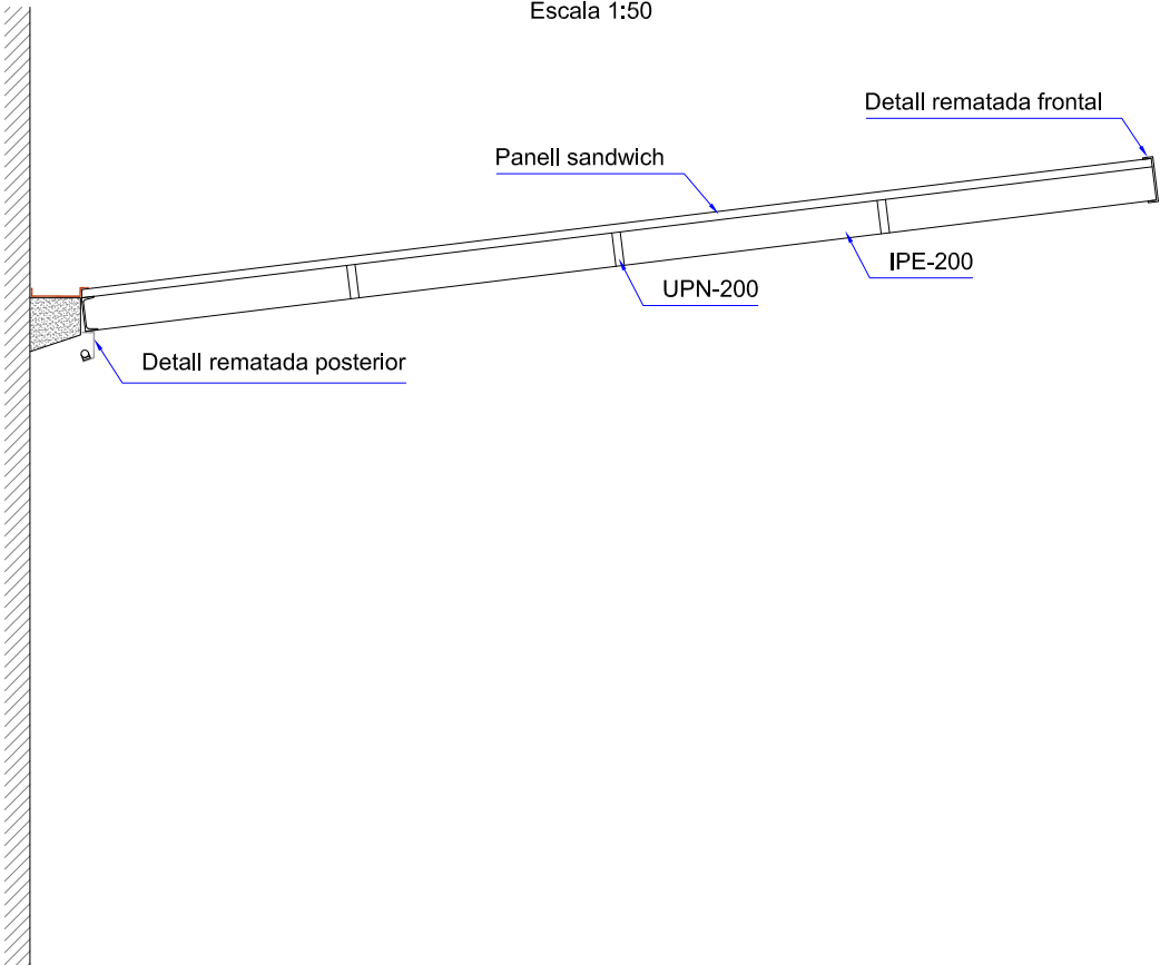
Secció marquesina Escala 1:50
