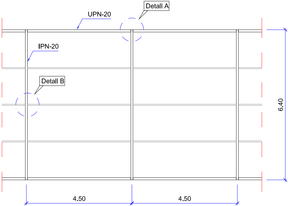
Mides estructura Escala 1:100
