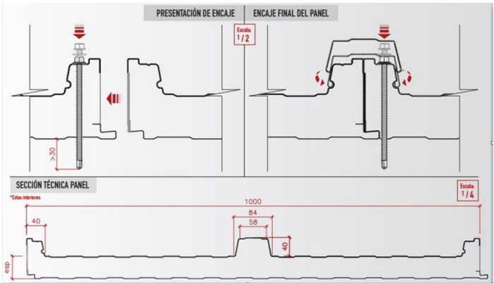
Detall muntatge frontal panell
