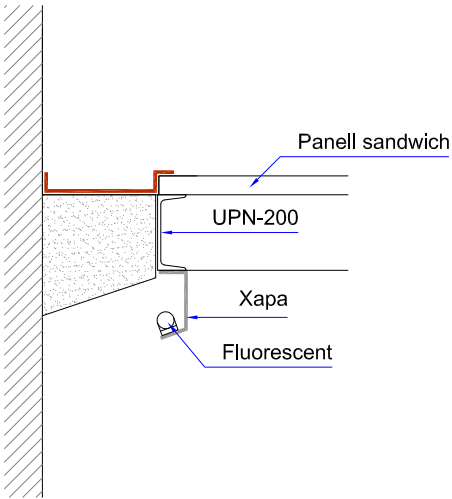
Rematada posterior Escala 1:20
