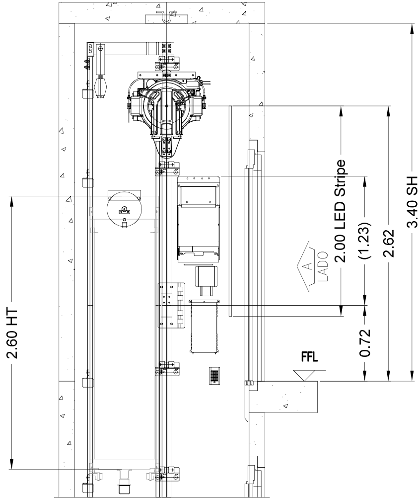
SECCIÓN A-A
