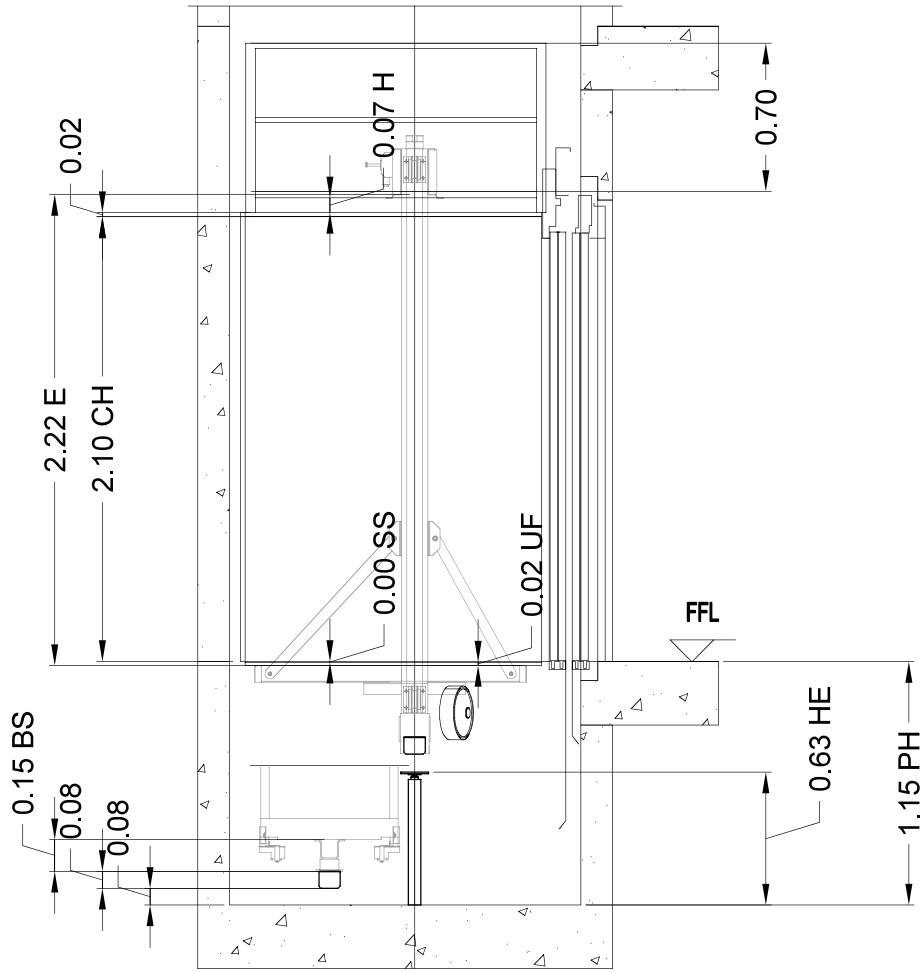
SECCIÓN A-A
