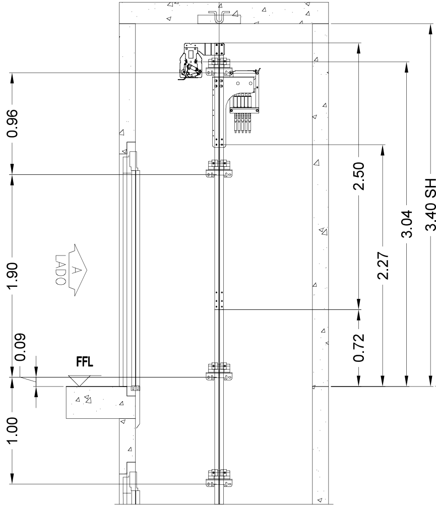
SECCIÓN B-B
