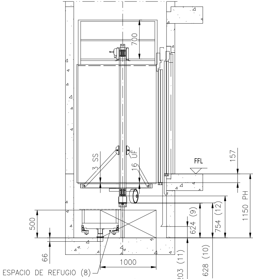
TOLERANCIAS FOSO Y HUÍDA sSECTION A-A Escala 1:45
