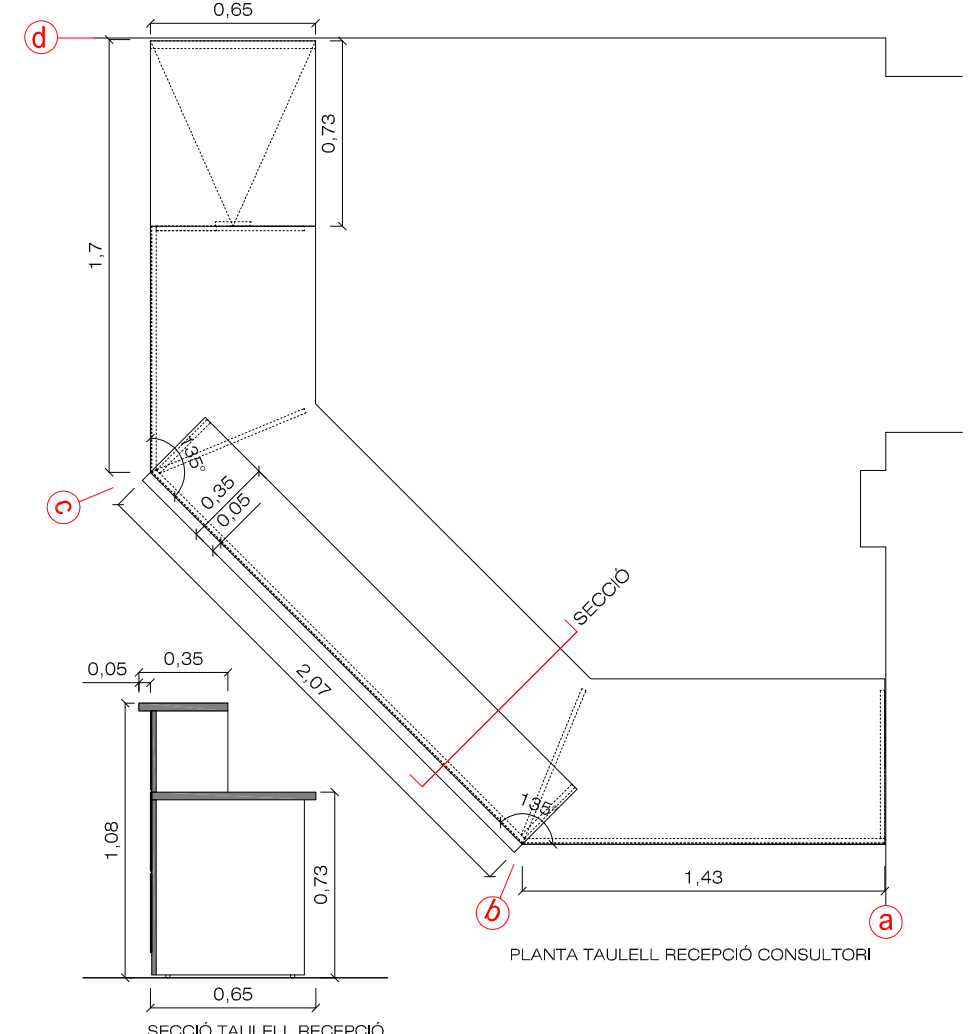
SECCIÓ TAULELL RECEPCIÓ
