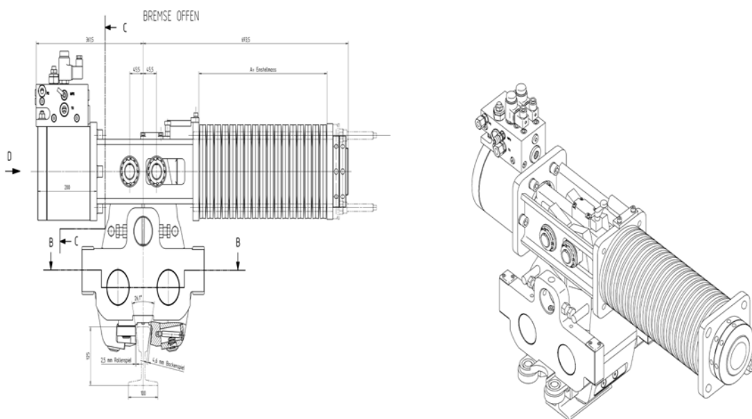
Imatge 2.- fre de carril
