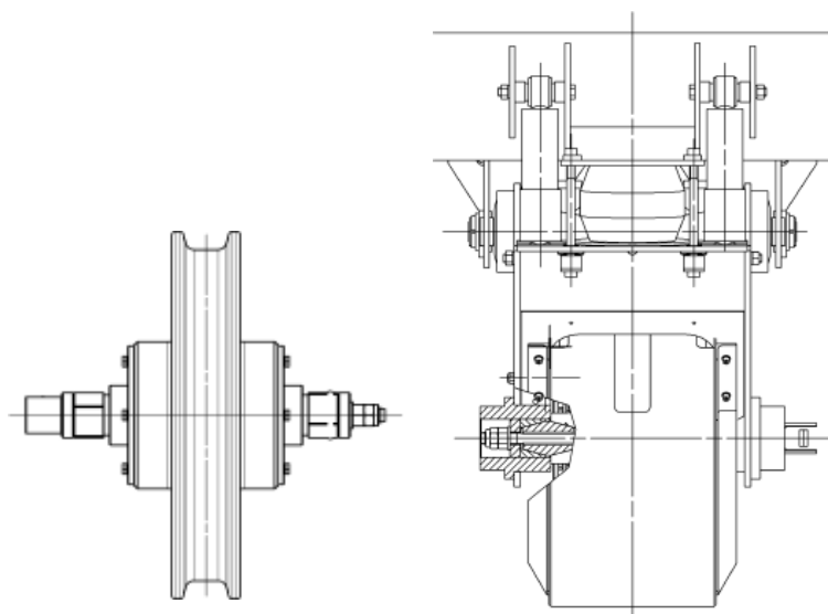
Imatge 1.- Roda de doble pestanya i roda plana.
