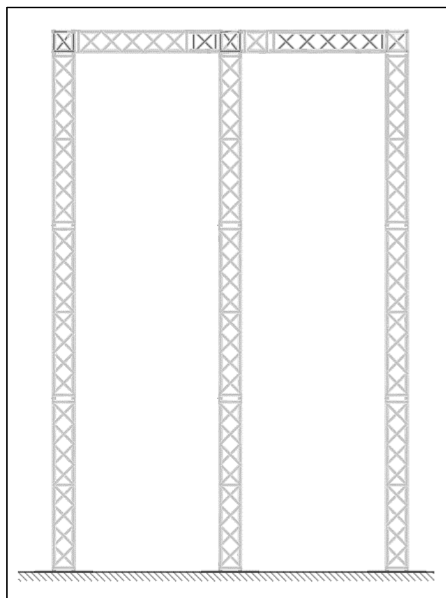
VISTA LATERAL
