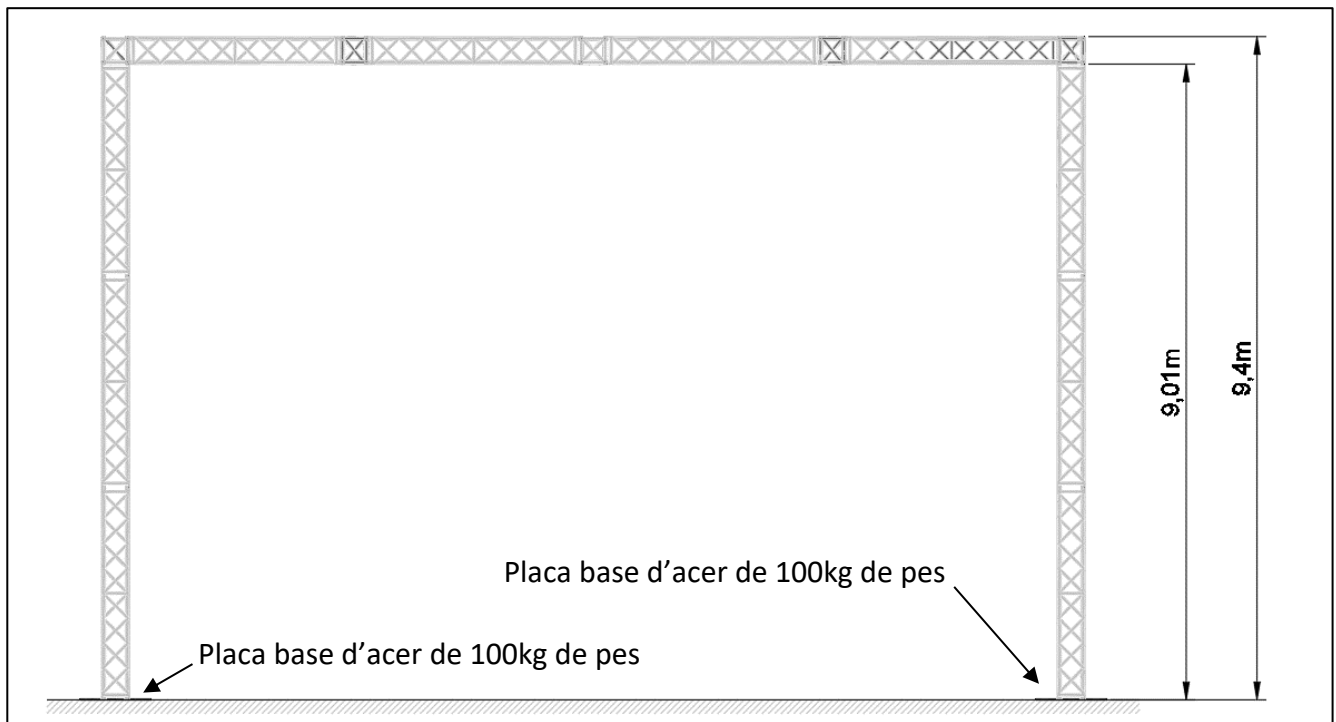
ALÇAT VISTA FRONTAL
