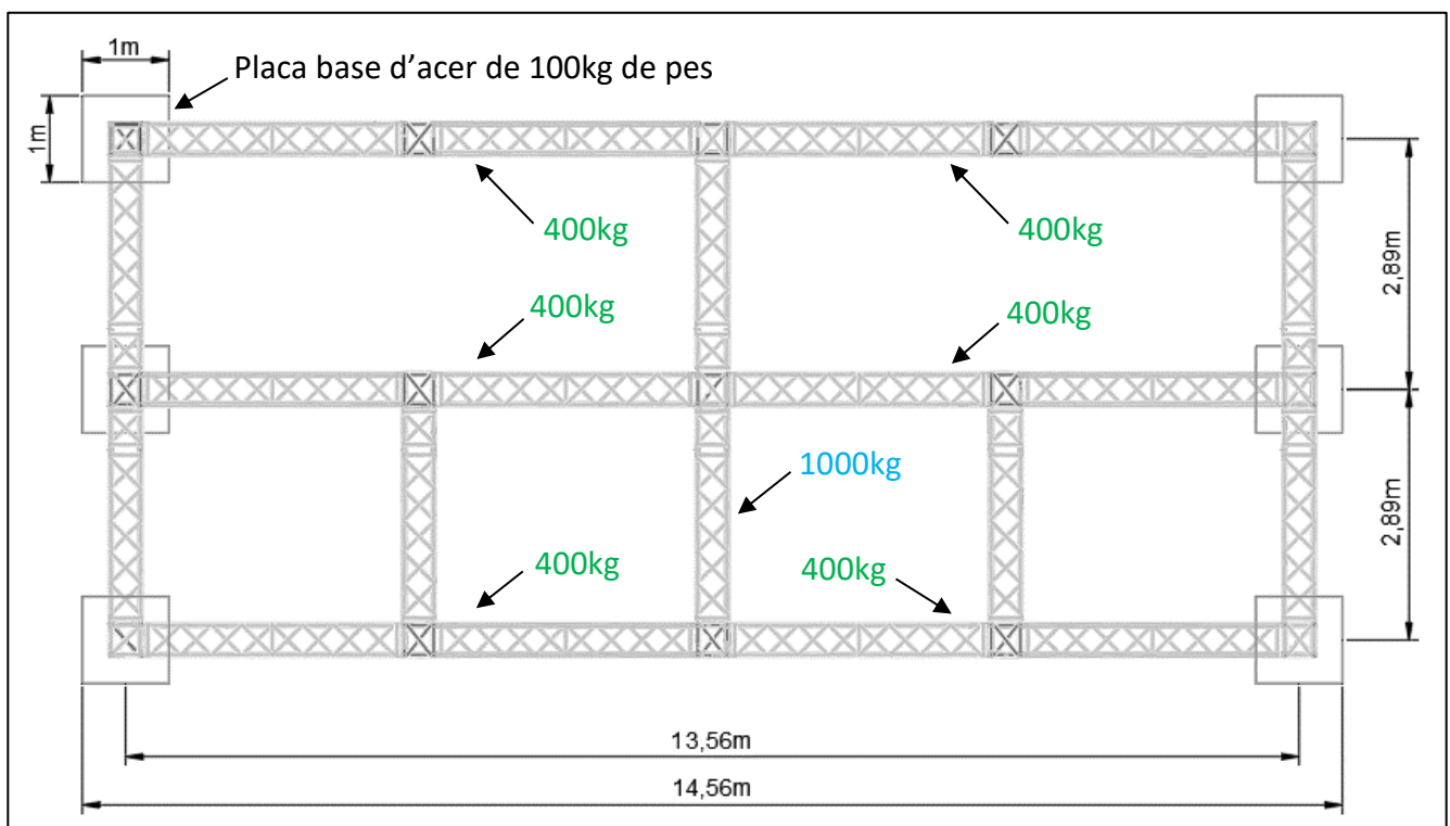
PLANTA
