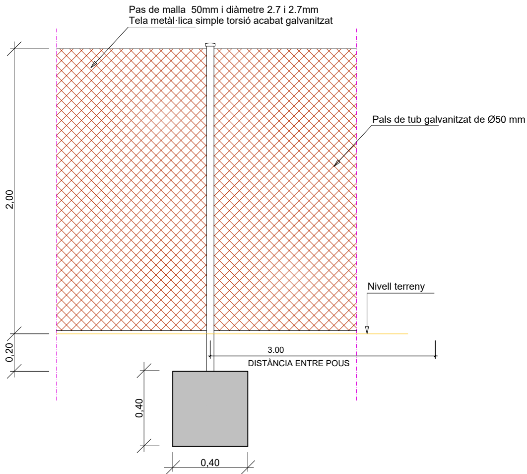
DETALL TANCA METÀL·LICA PERÍMETRE
