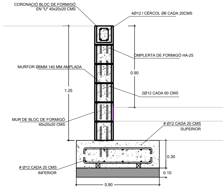
SECCIÓ MUR 2 1/25
