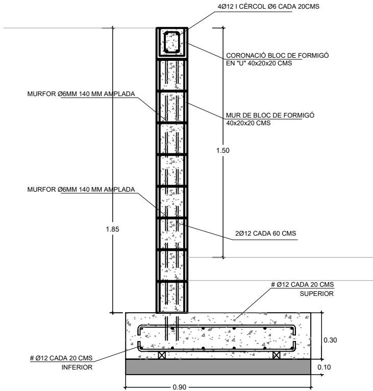
SECCIÓ MUR 1 1/25
