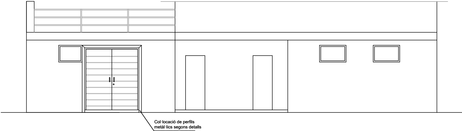
ALÇAT FRONTAL PROPOSTA
