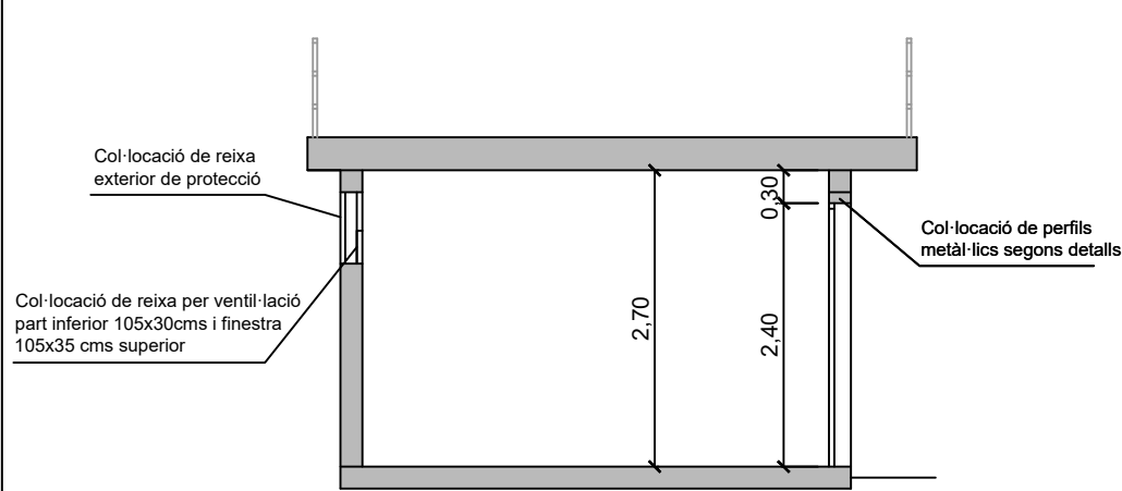
SECCIÓ PROPOSTA
