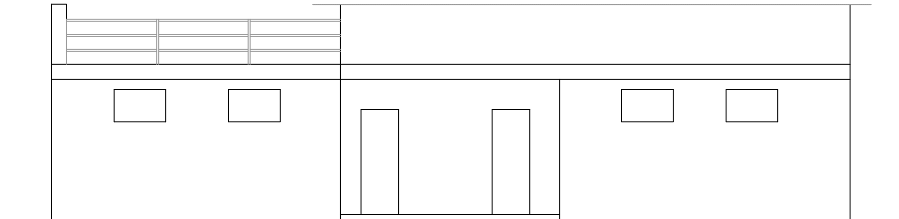
ALÇAT FRONTAL
