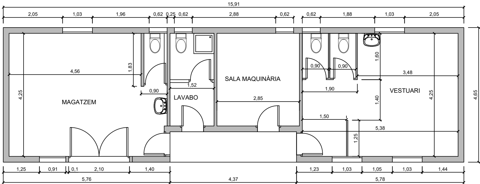
PLANTA PROPOSTA COTES
