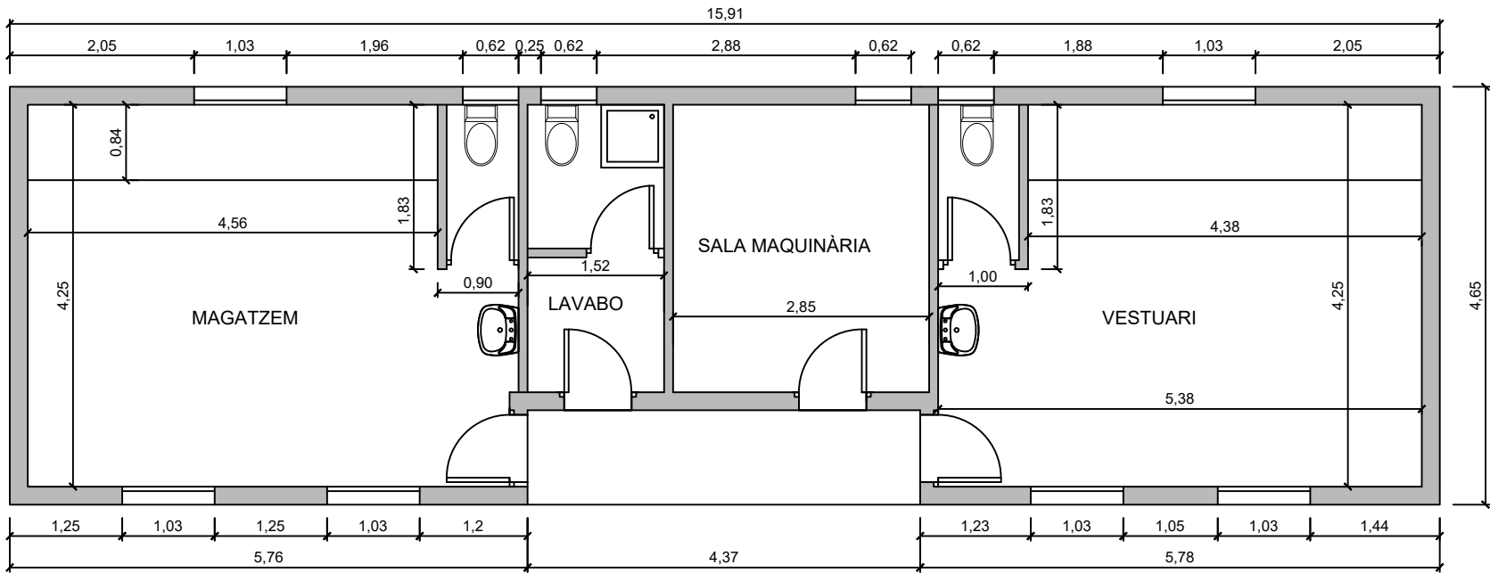
PLANTA ESTAT ACTUAL
