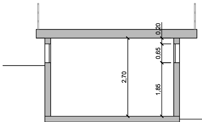
SECCIÓ ESTAT ACTUAL
