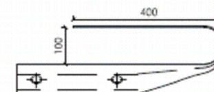
TOPE FINAL DE BARRERA ESTANDAR (abellente) ESCALA 1:10
