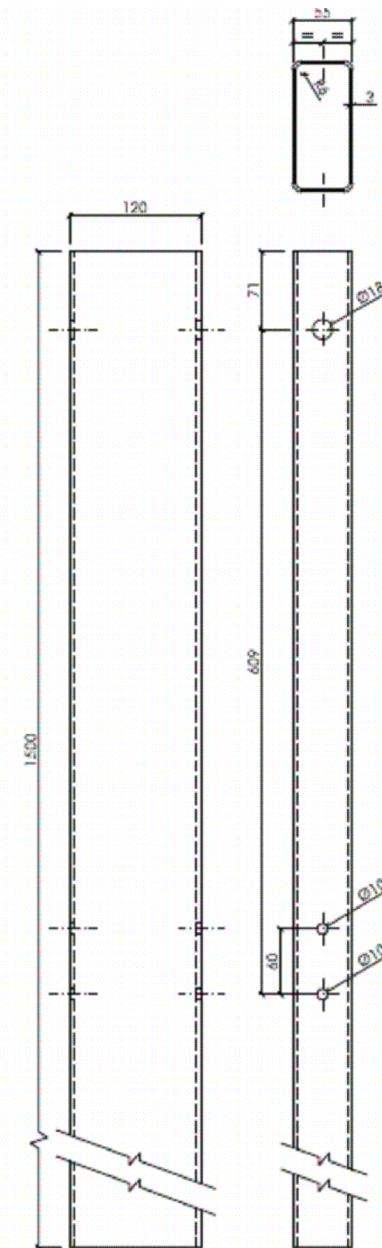
POSTE TUBULAR 1,5m. ESCALA 1:5
