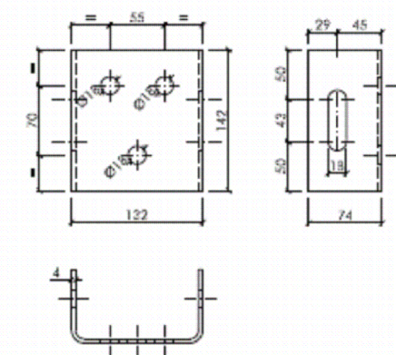
CONECTOR ESCALA 1:5
