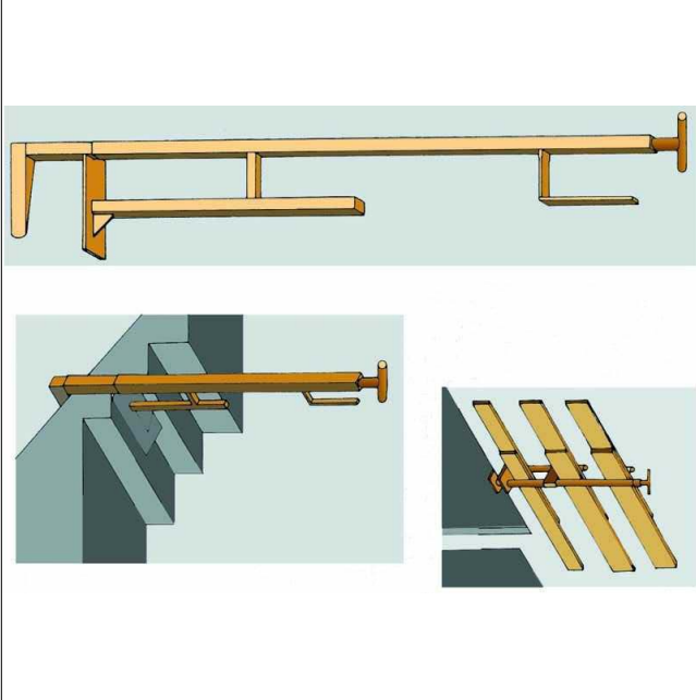
Baranes de seguretat Amb sergent 1
