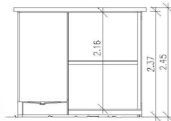
SECCIÓ A-B
