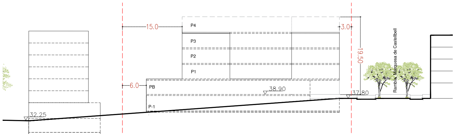
SECCIÓ A-A'
