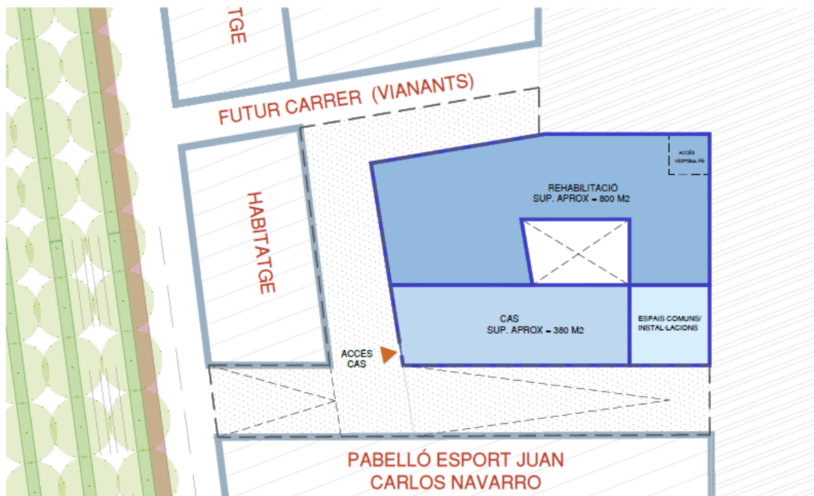
PLANTA -1 (ACCÉS RAMBLA MAJOR)
