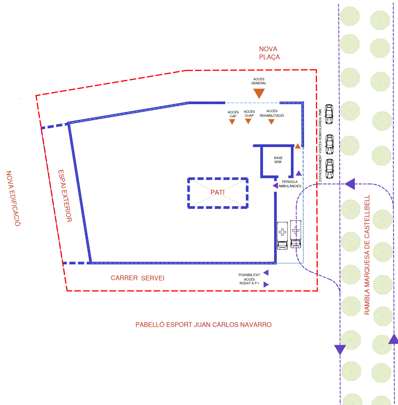
PROPOSTA ESQUEMÀTICA PLANTA BAIXA
