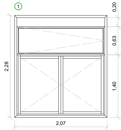
Finestra corredissa amb part fixa
