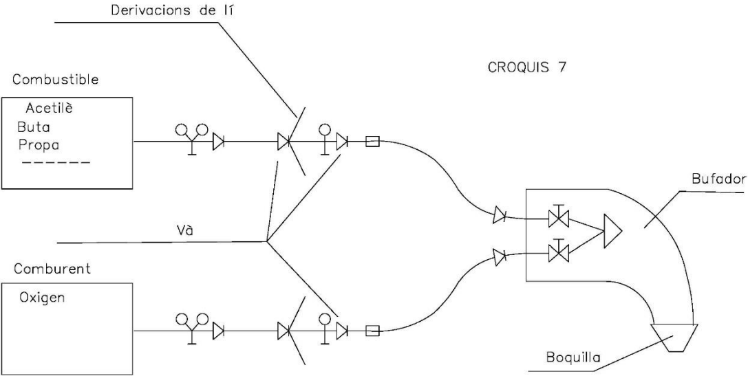
ESQUEMES DE COMPONENTS D'UNA INSTAL·LACIÓ OXITALLADA
