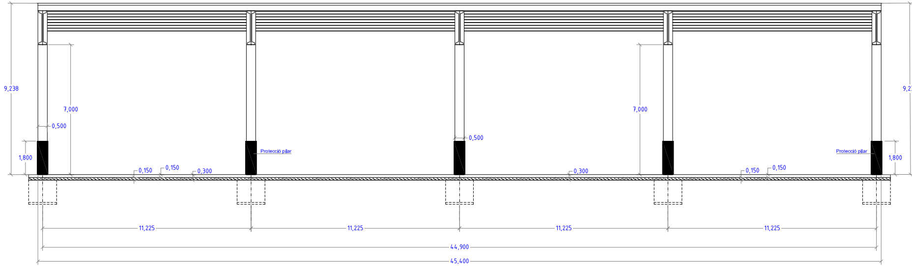
SECCIÓ LONGITUDINAL
