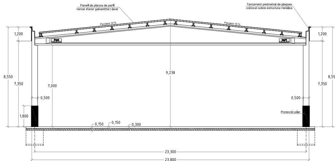
ALÇAT NORD
