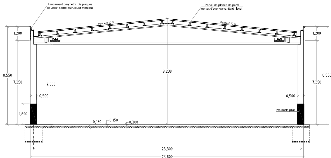
ALÇAT SUD
