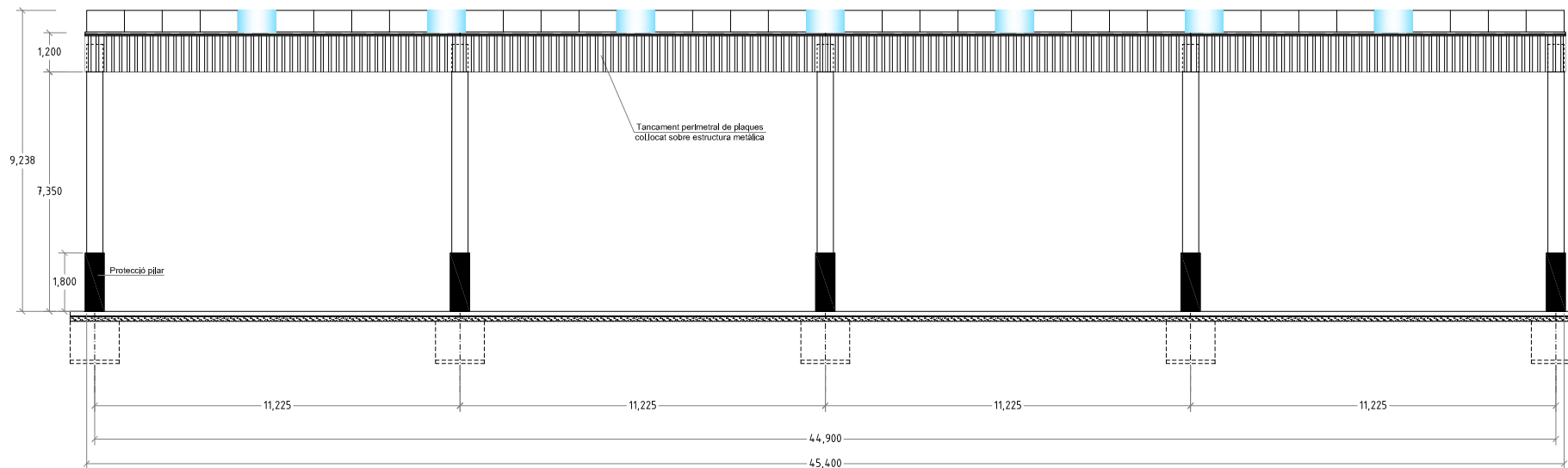
ALÇAT OEST
