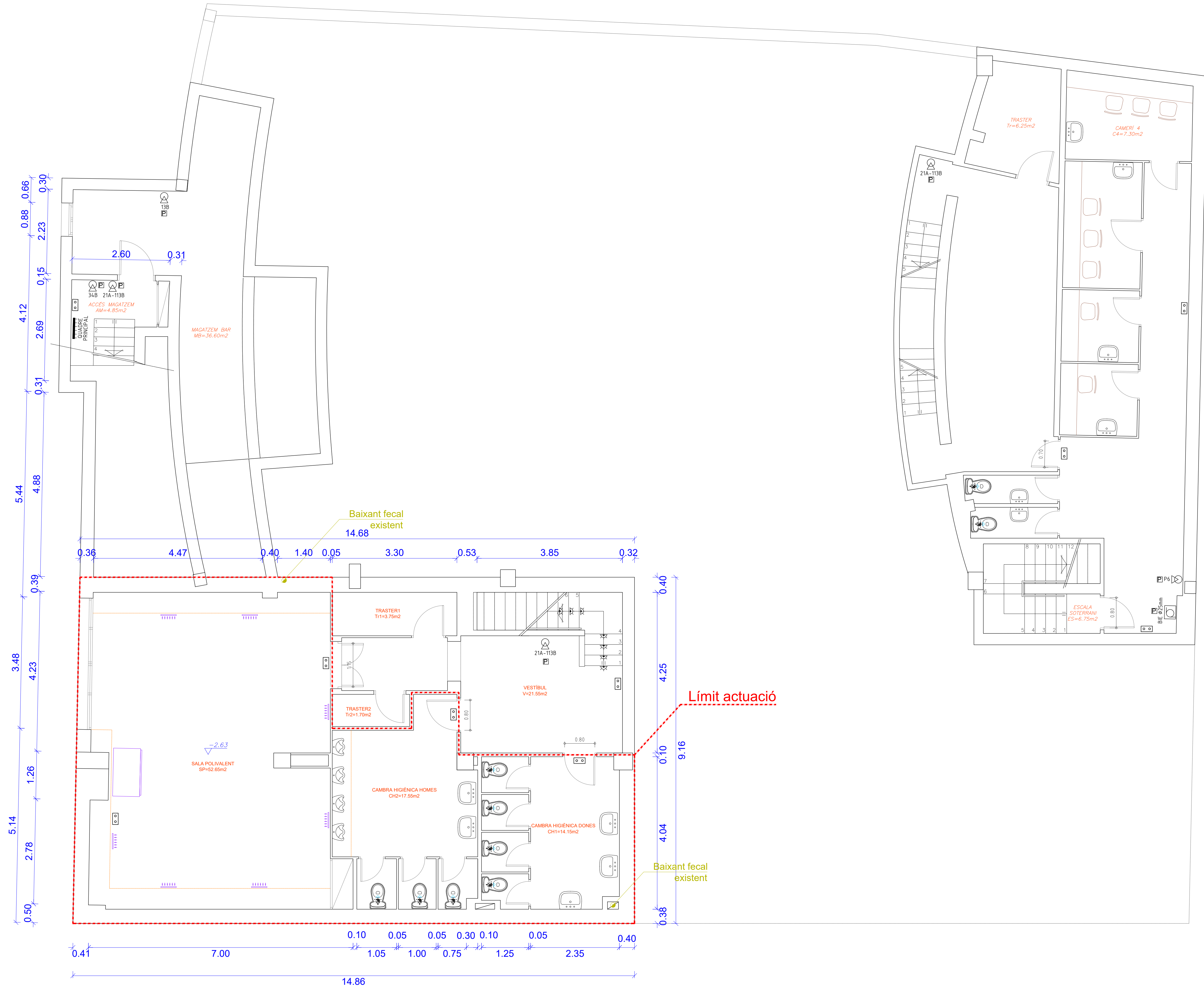
PLANTA SOTERRANI
