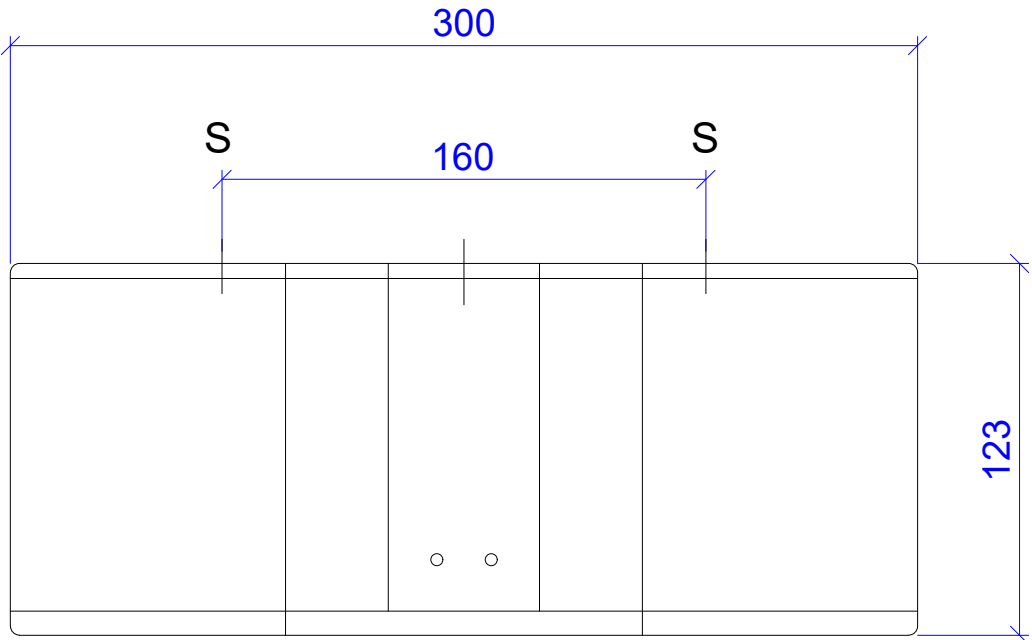
S - punts d'ancoratge a paret
