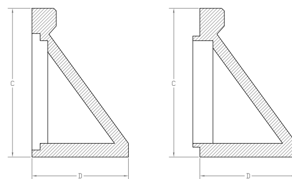
BROQUET PER A DESGUAS DE CANONADA s/e
