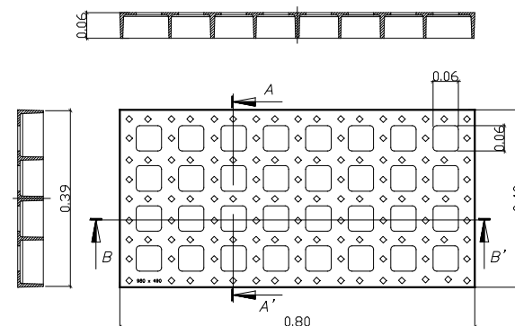
REIXA EMBORNAL e: 1/10
