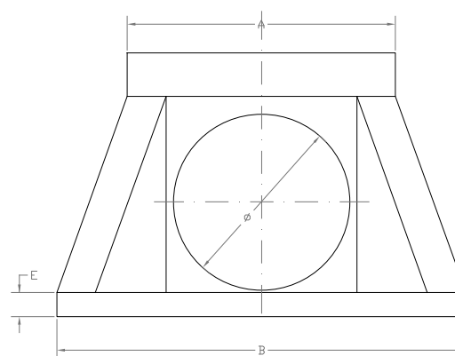
ALÇAT
