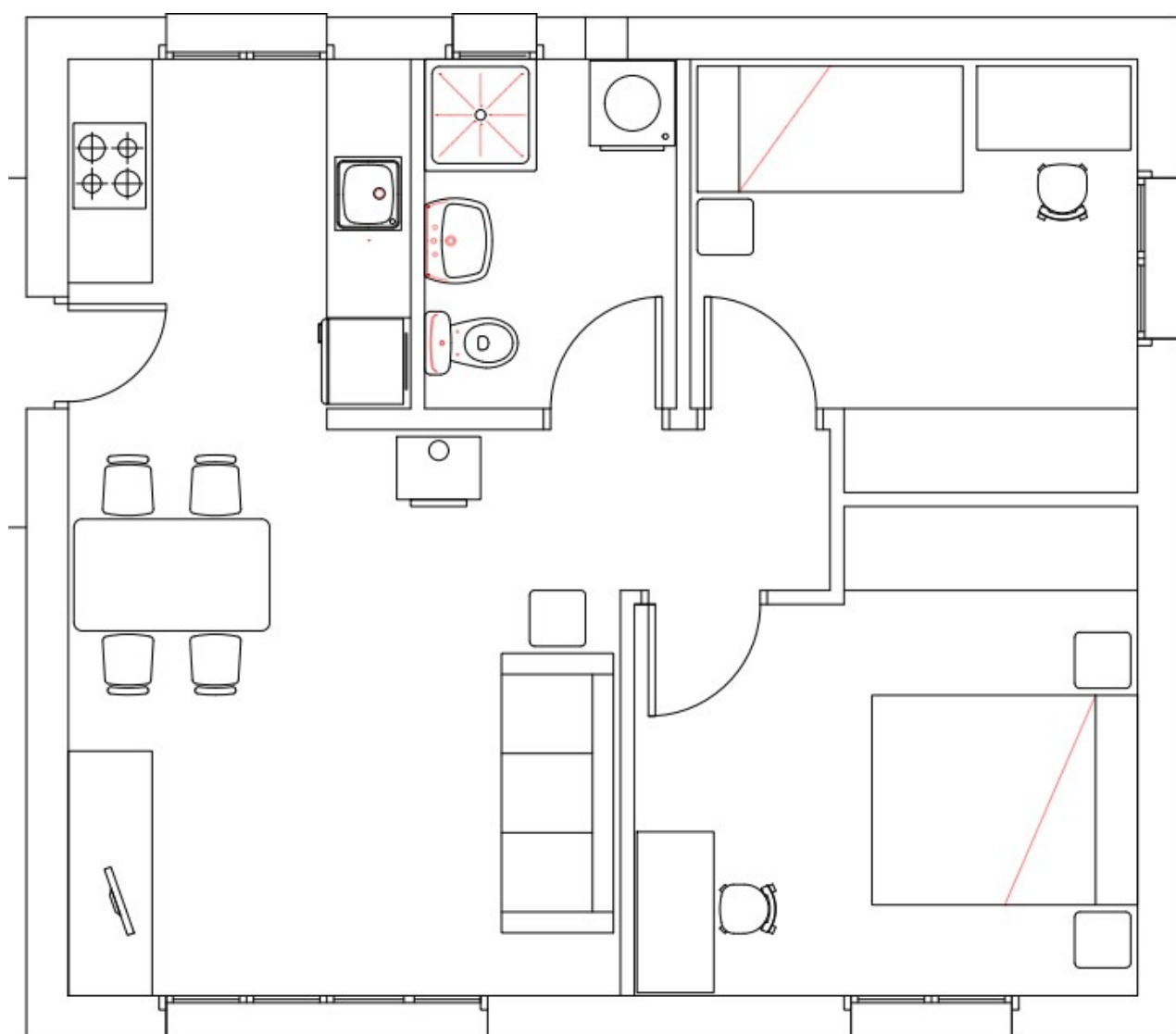
Proposta planta distribució E.- 1:50
