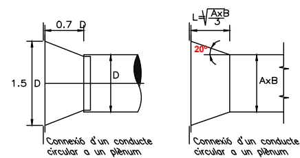
Detalls de connexions (mides de mm)
