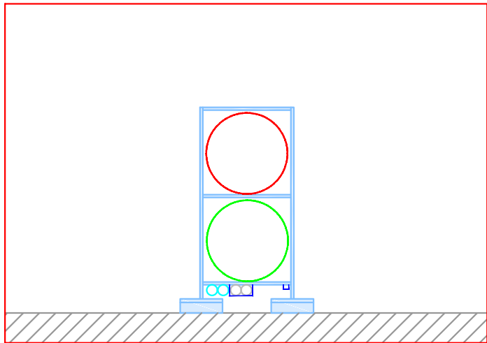
DETALL SUBESTRUCTURA DE SUPORTACIÓ
