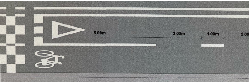
DETALLS TIPUS SENYALITZACIÓ HORIZONTAL EN CARRIL BICI
