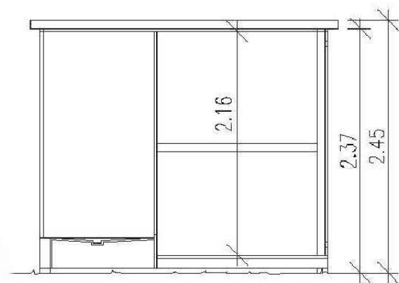
SECCIÓ A-B
