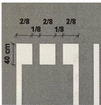
DETALLS TIPUS SENYALITZACIÓ HORIZONTAL EN CARRIL BICI
