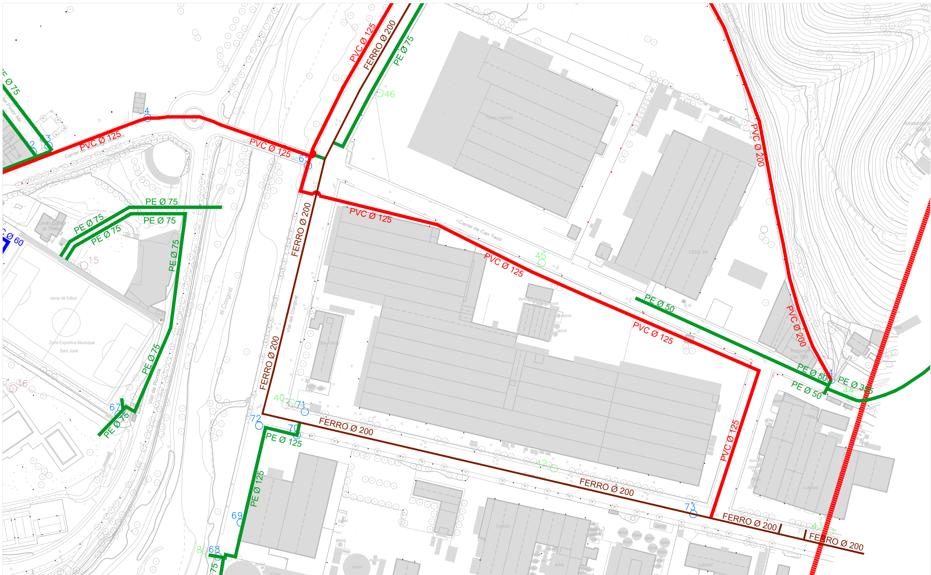
PLÀNOL DE CANALITZACIONS D'ABASTAMENT D'AIGUA (canalitzacions per vorera)
