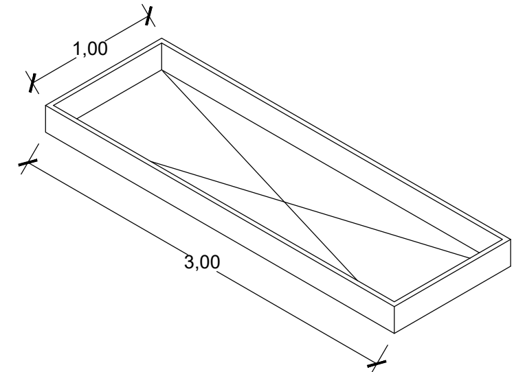
Escossell 300x100cm metàl.lic d'acer corten amb platabanda de 20cmm d'amplada i 5mm de gruix.
