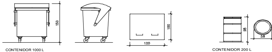
CONTENIDOR 1000 L
