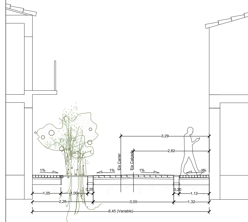
Secció tipus
