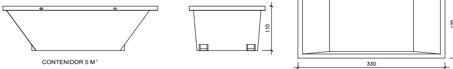
CONTENIDOR 5 M 3
