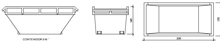
CONTENIDOR 9 M 3
