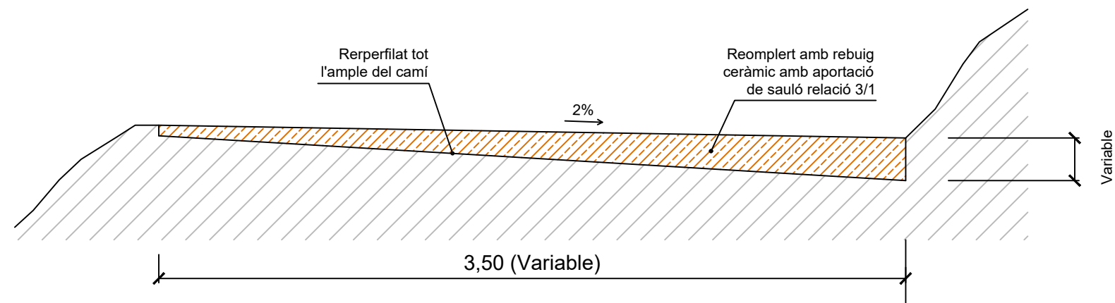
SECCIÓ TIPUS 2
