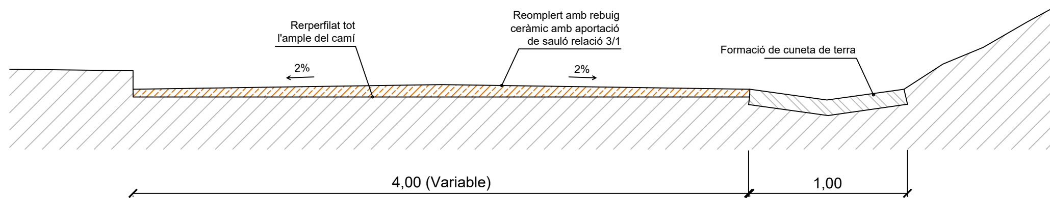
SECCIÓ TIPUS 1
