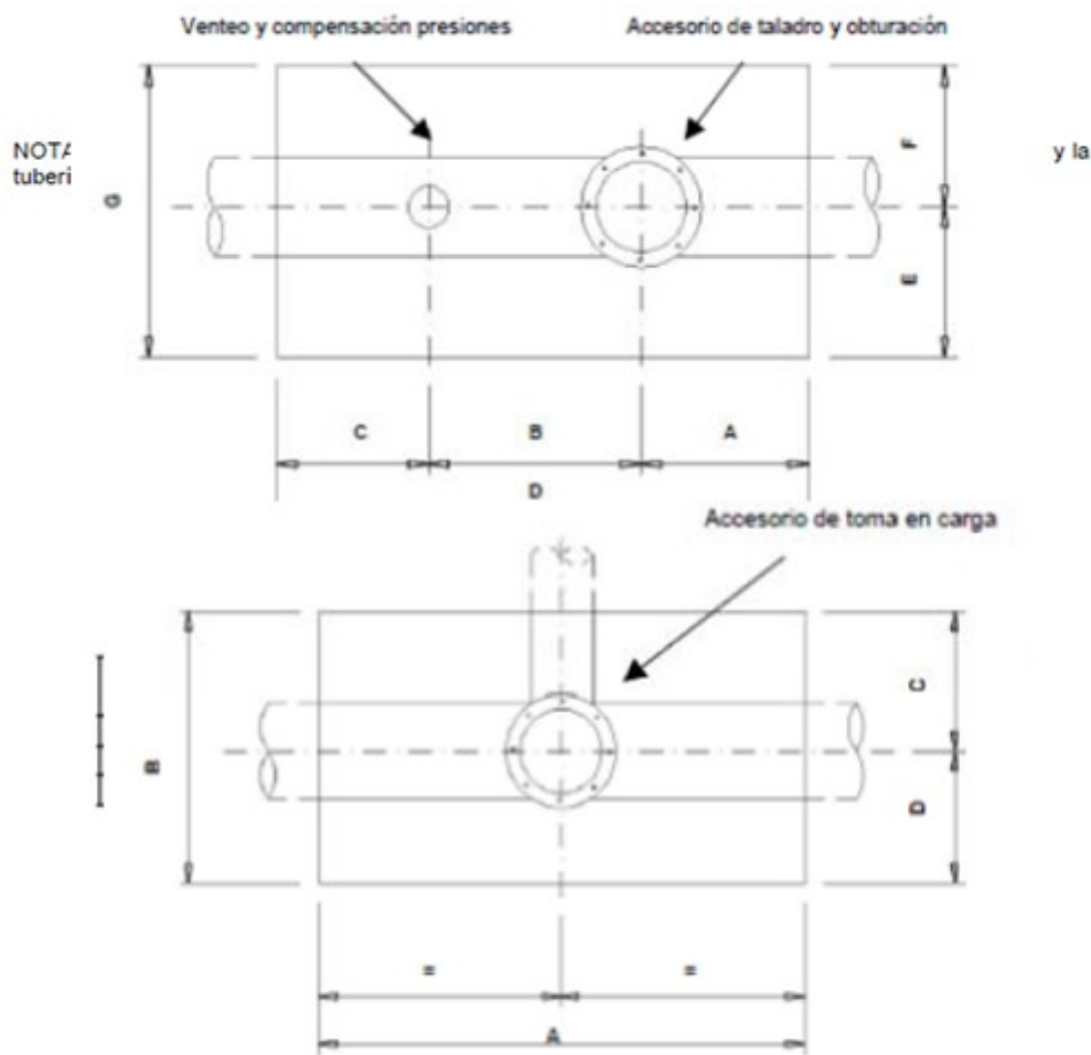
Dimensiones de zanjas en derivaciones
