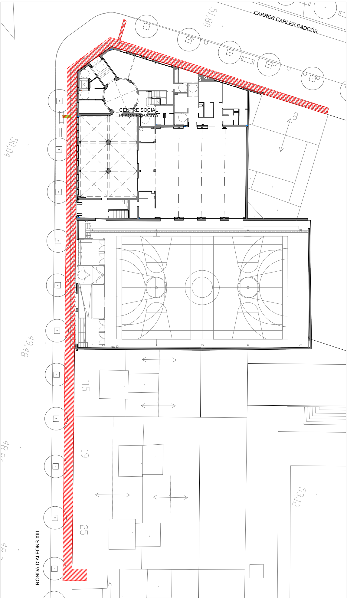
EMPLAÇAMENT E 1:400
