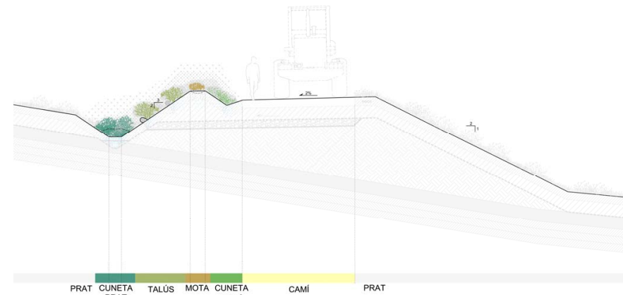
Secció tipus dels treballs de plantació al camí de manteniment.
