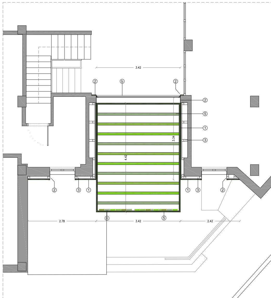
PLANTA PRIMERA. ACCÉS CARRER GRUP ESCOLAR
