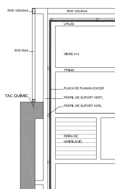
DETALL 1 - ESC: 1/25
