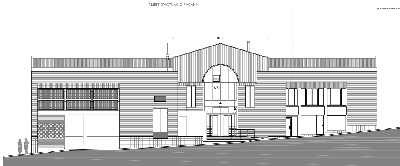
FAÇANA CARRER GRUP ESCOLAR
