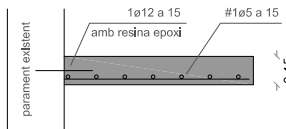
SOLERES esc: 1/25
