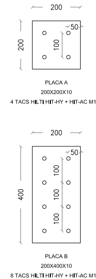
DETALLS PLAQUES ESC: 1/10
