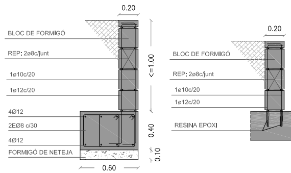
MUR A esc: 1/25
