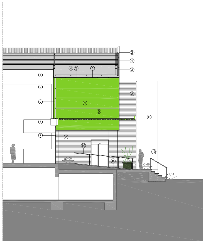
SECCIÓ ACCÉS CARRER CAMPINS
