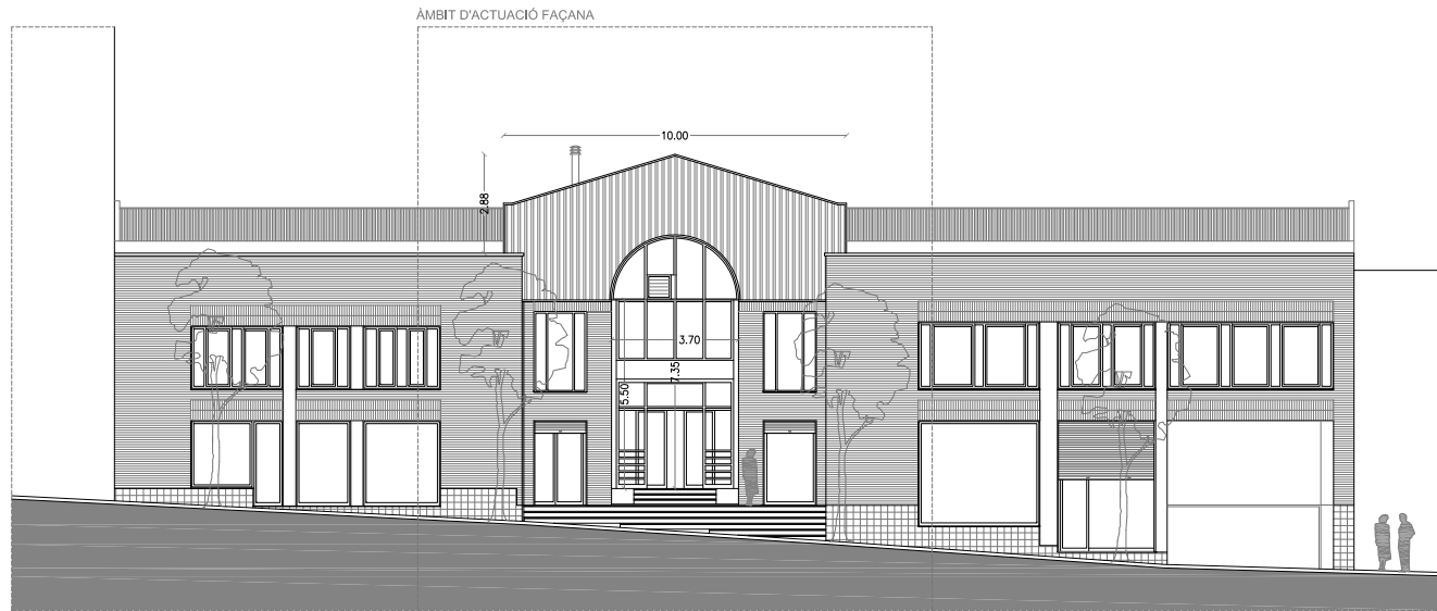
FAÇANA CARRER CAMPINS
