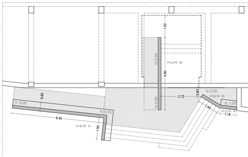
FNAMENTS esc: 1/100
