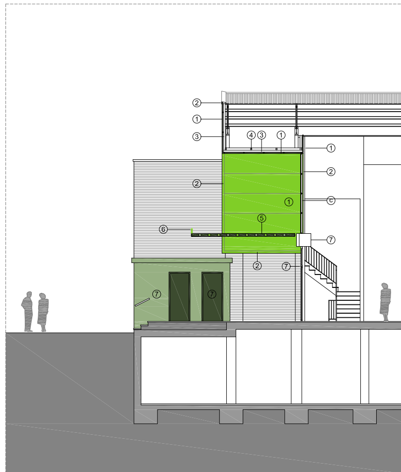
SECCIÓ ACCÉS CARRER GRUP ESCOLAR
