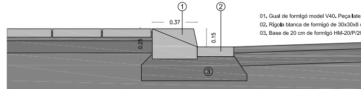
GUAL VEHICLES V40 - PEÇA LATERAL
