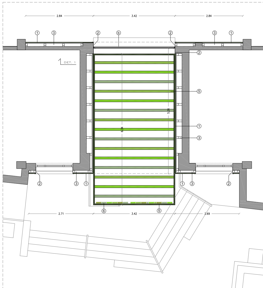
PLANTA PRIMERA. ACCÉS CARRER CAMPINS
