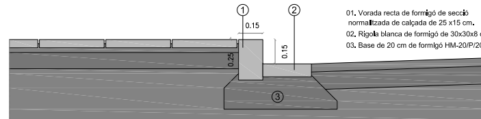
VORADA RECTA
