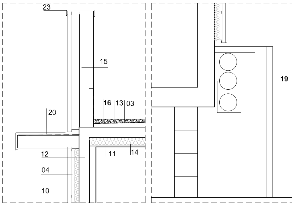
DETALL D02
