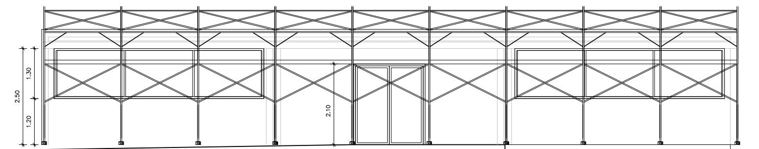
ALÇAT BASTIDA
