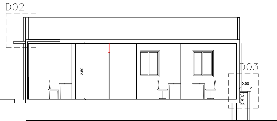
SECCIÓ B-B'
