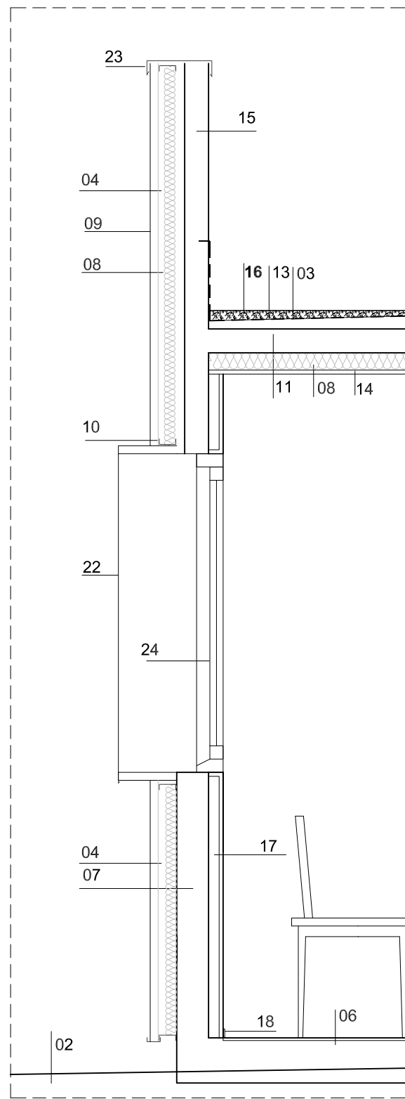
DETALL D01
