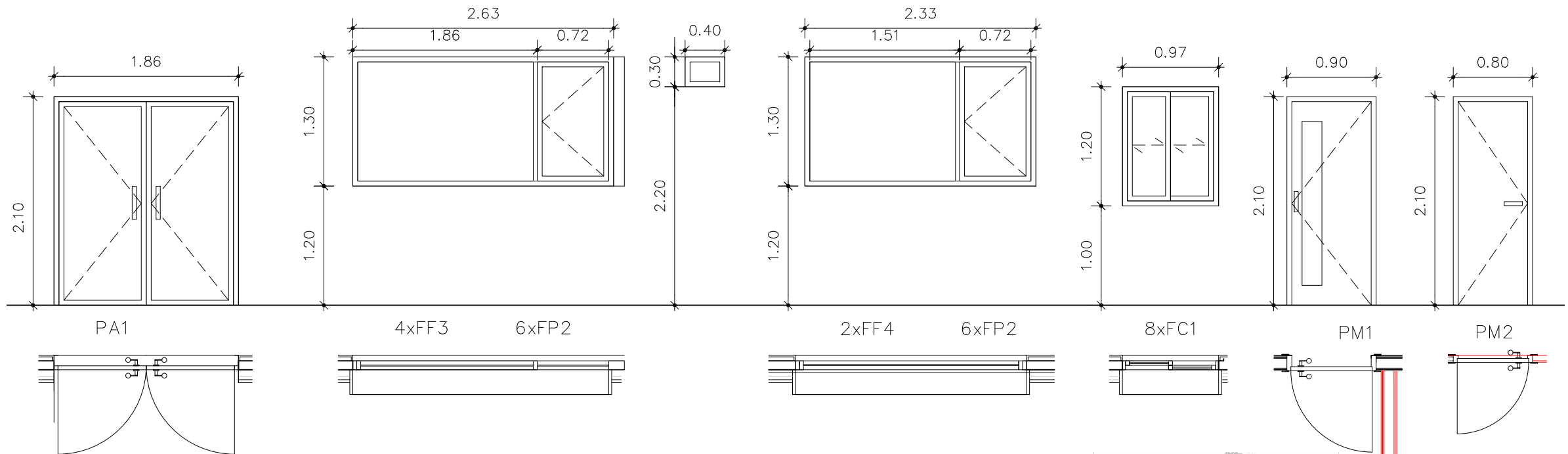
FUSTERIA
