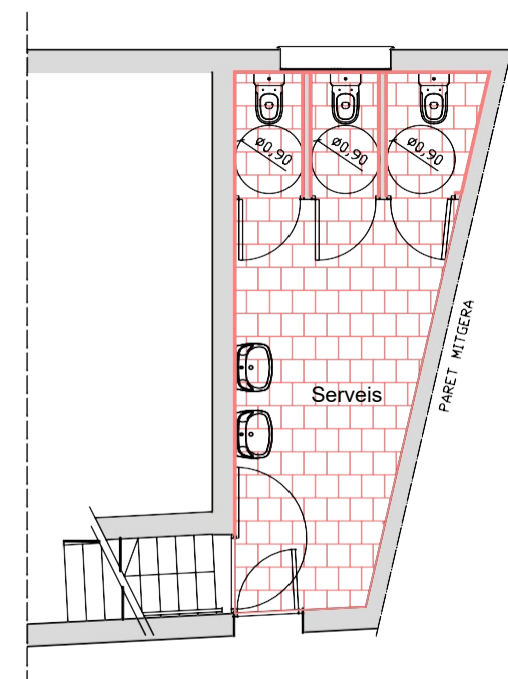
PLANTA SEMISOTERRANI
