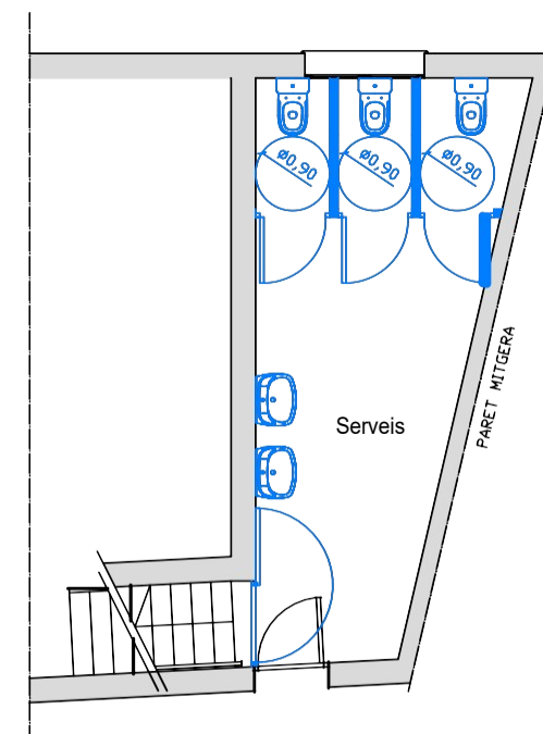
PLANTA SEMISOTERRANI
