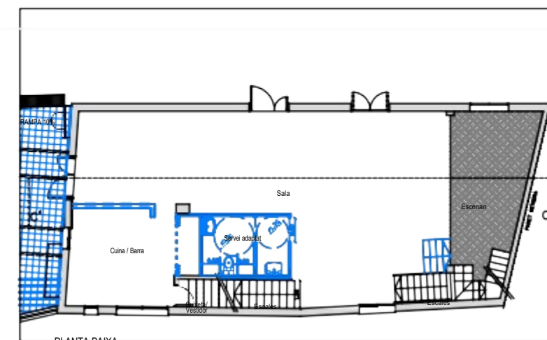
PLANTA BAIXA
