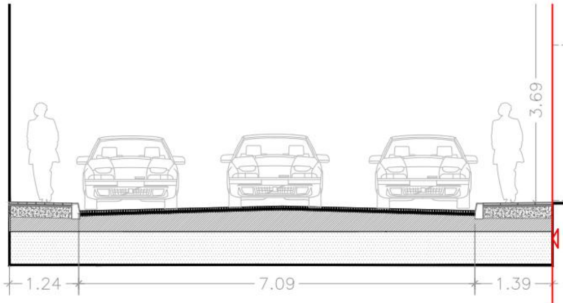
Imatge 3 Secció carrer
