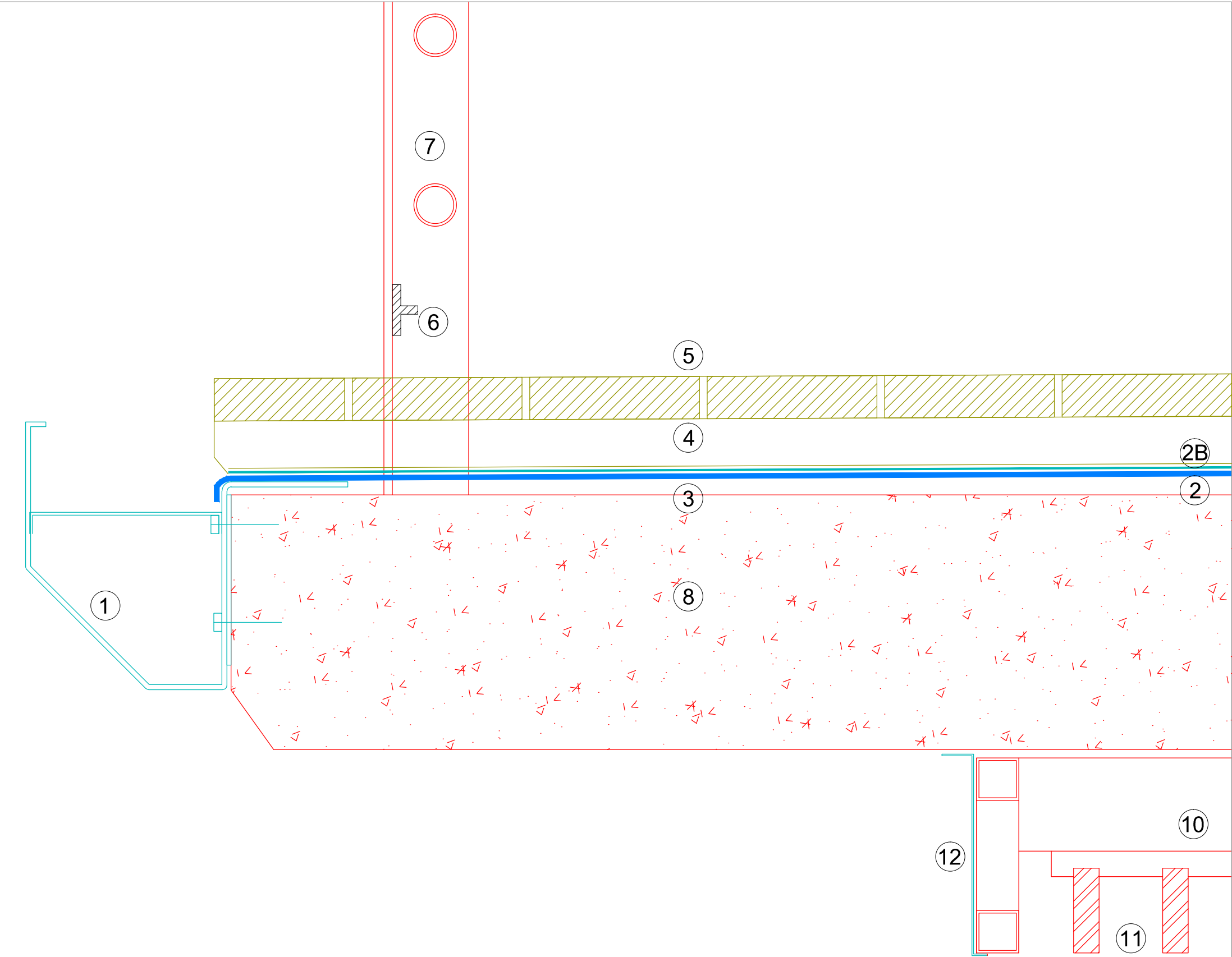
DETALL VOLADIU SOBRE ESCALES
