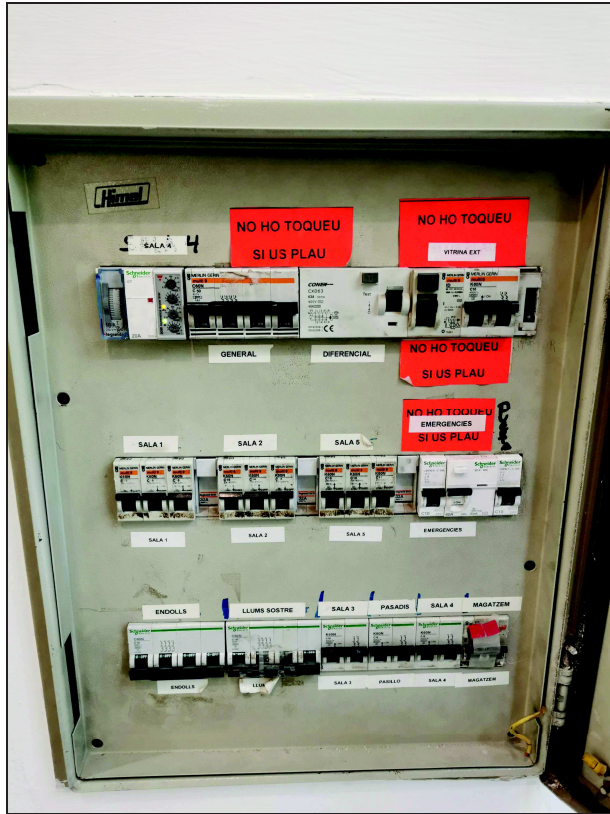
Subquadre elèctric sala d'exposicions
