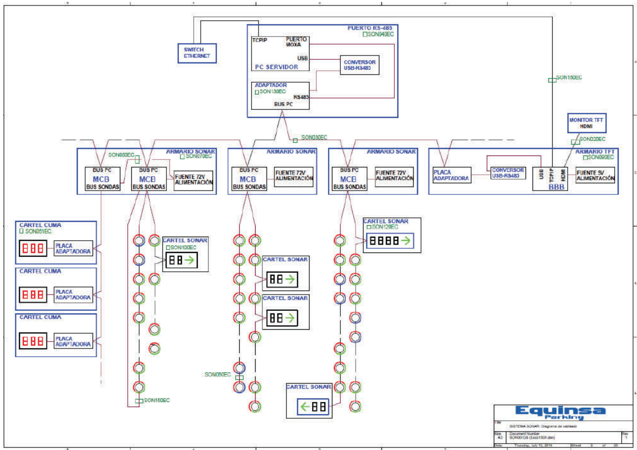
Esquema de cableado General
