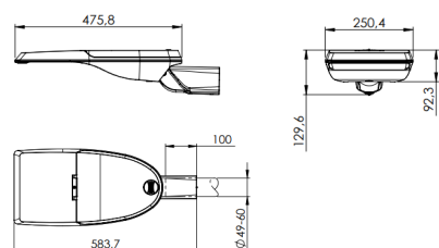
Fijación lateral \varnothing 49/60 mm (SE2)
