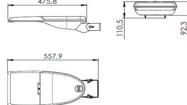
Fijación mural. Incorpora horquilla (FM1)
