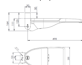
Fijación a techo. Incorpora horquilla para fijación directa a techo (FT1)
