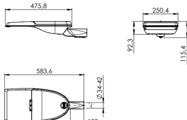
Fijación lateral \varnothing 34/42 mm (SE1)
