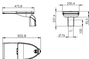
Fijación vertical \varnothing 76 mm (PT1)
