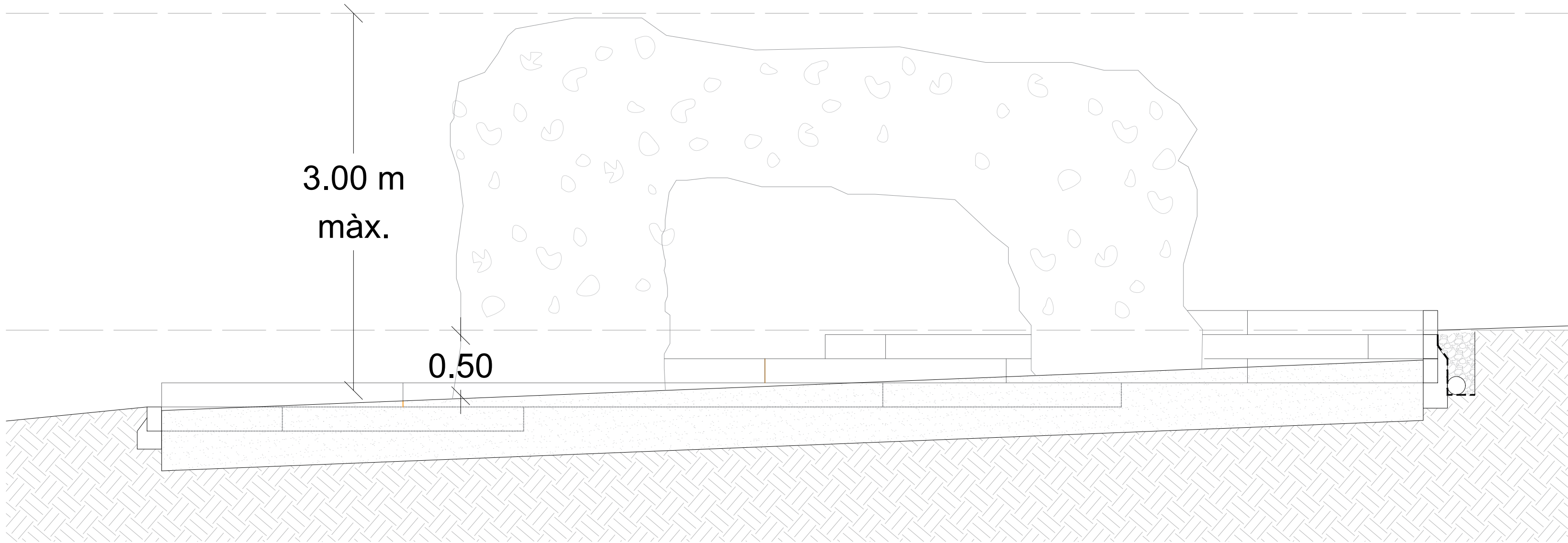
SECCIÓ LONGITUDINAL ROCÒDROM
