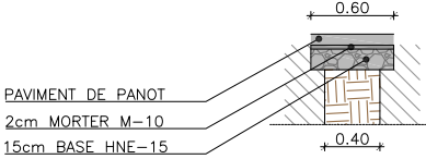
DETALL RASA EN VORERA E: 1/60
