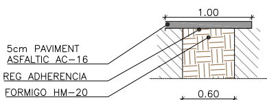
DETALL RASA EN CALÇADA E: 1/60
